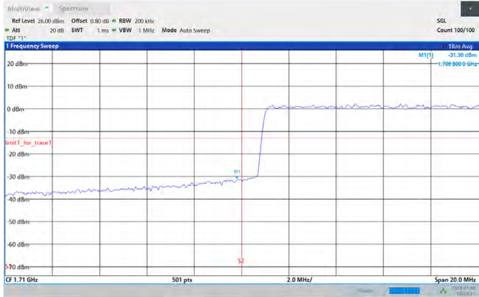
Band66-20MHz-QPSK-132572-1RB#99
