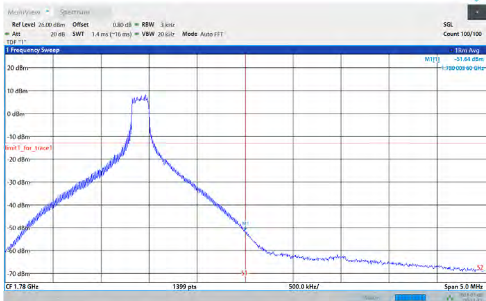
Band66-20MHz-QPSK-132572-100RB#0
