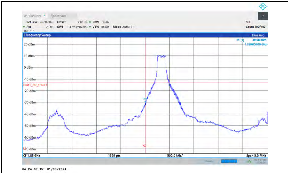
Band2-5MHz-QPSK-18625-25RB#0
