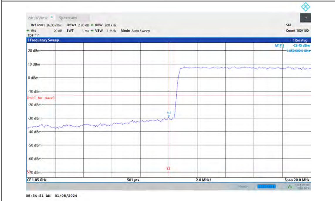
Band2-15MHz-16QAM-19125-1RB#74
