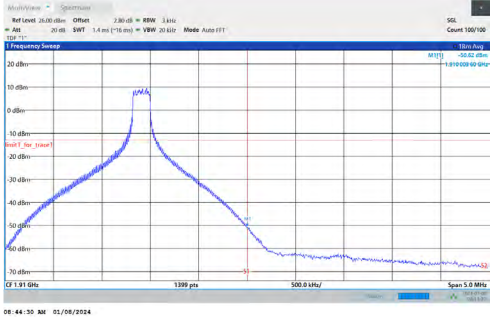
Band2-20MHz-QPSK-19100-100RB#0
