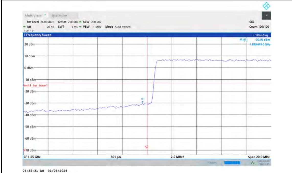
Band2-15MHz-64QAM-19125-1RB#74
