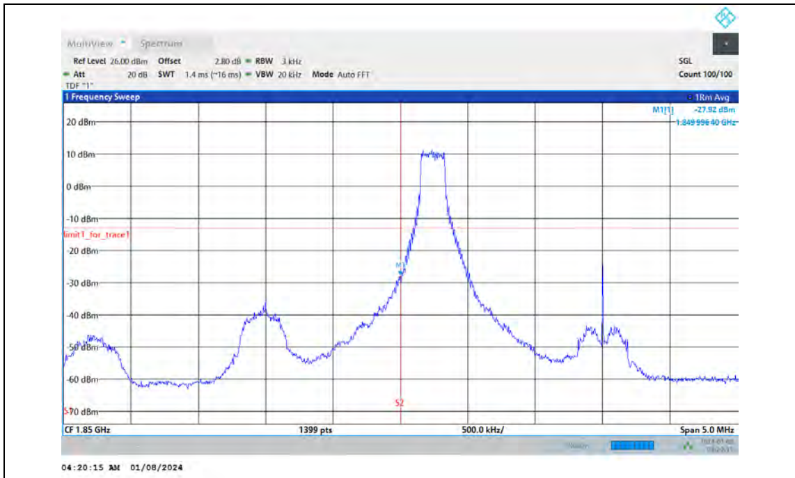
Band2-3MHz-QPSK-18615-15RB#0
