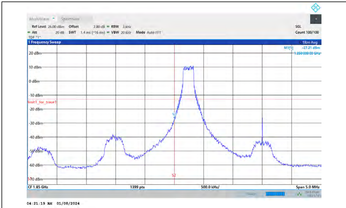
Band2-3MHz-16QAM-18615-15RB#0
