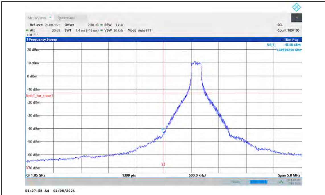
Band2-10MHz-QPSK-18650-50RB#0
