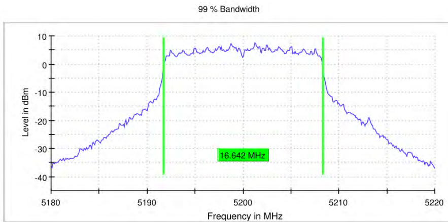
11A_Ant0_5200
