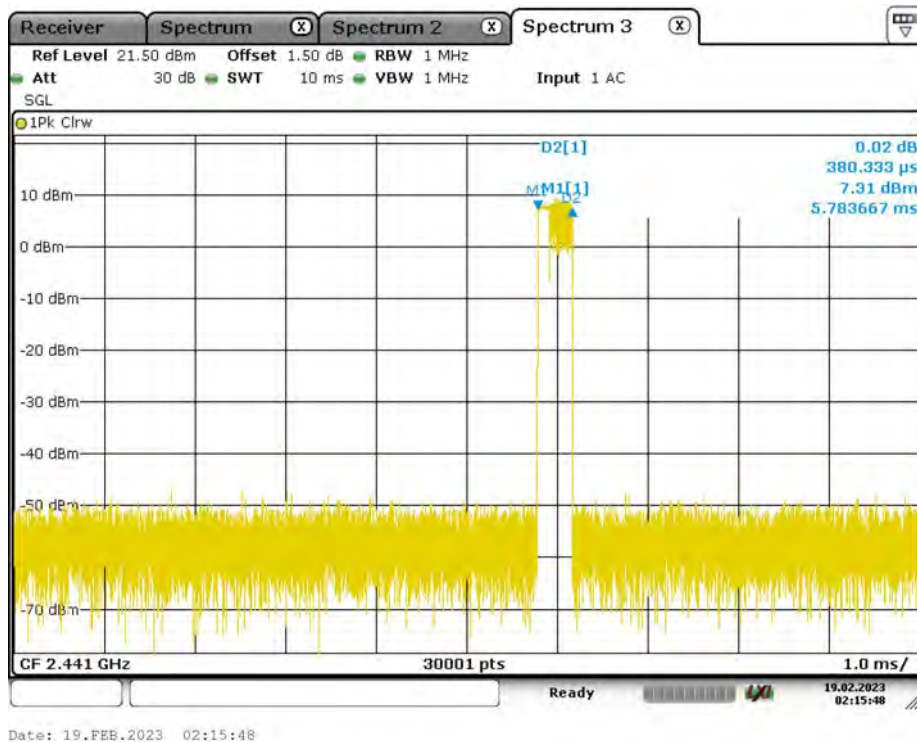
3DH1_Ant1_Hop
