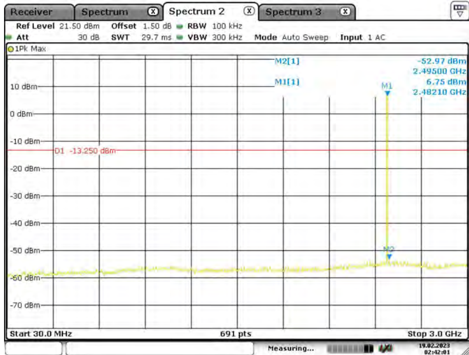
DH5_Ant1_2480_30~3000
