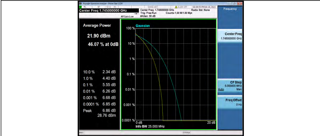
Band66-20MHz-QPSK-132572-1RB#0
