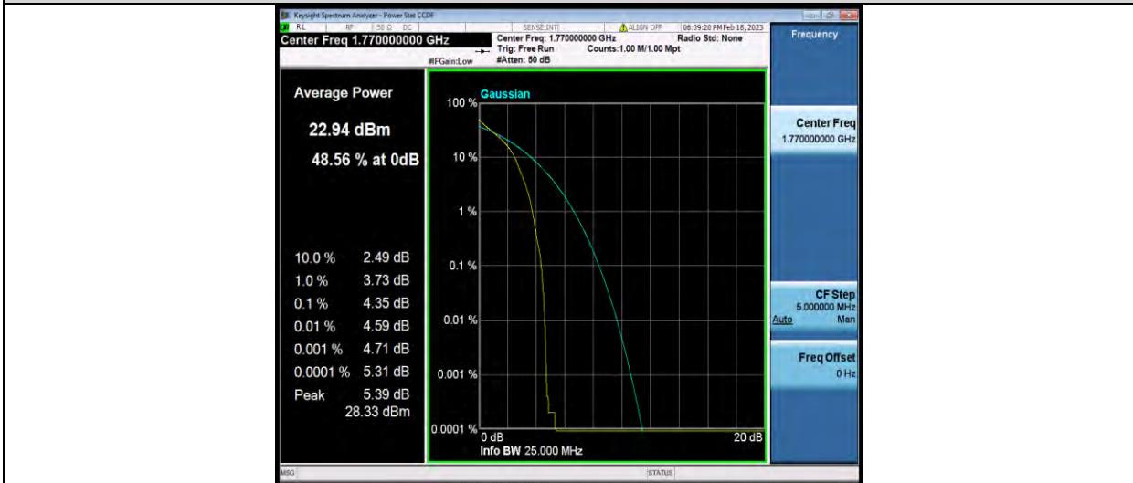
Band66-20MHz-QPSK-132572-100RB#0
