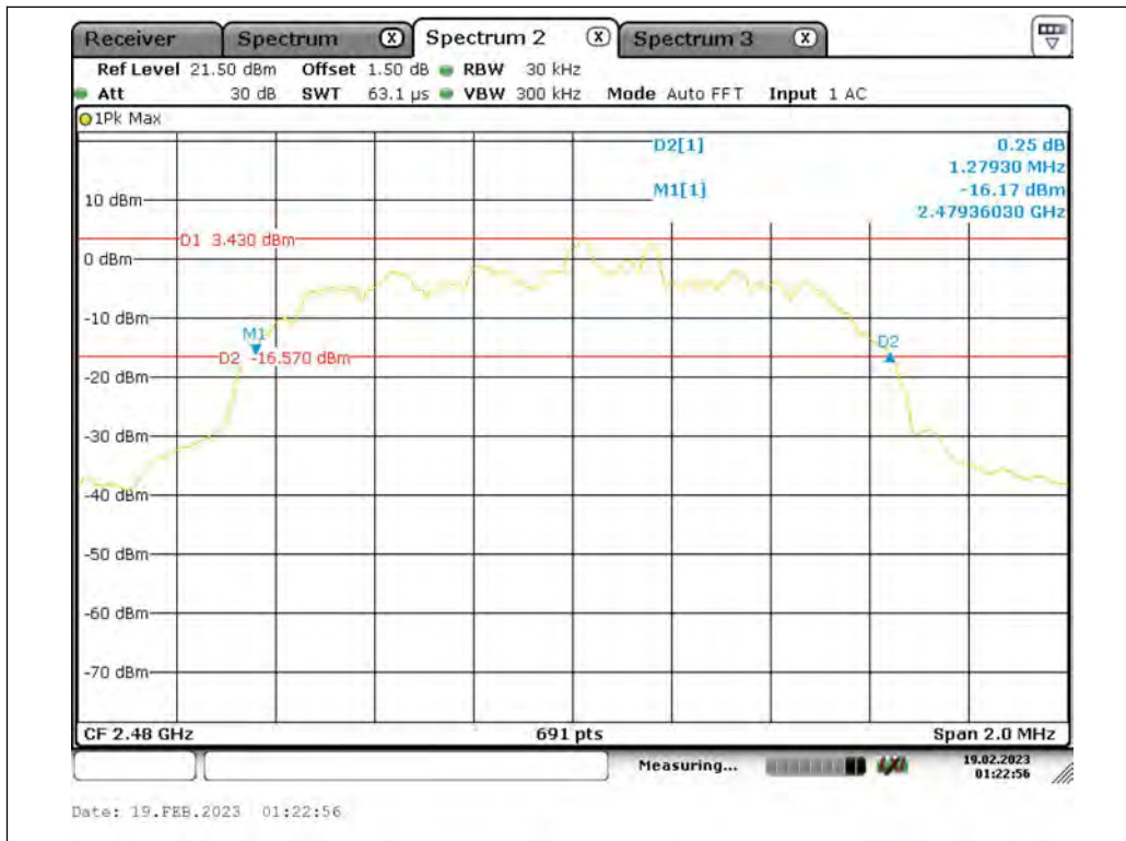
2DH5_Ant1_2480
