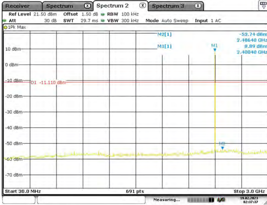
DH5_Ant1_2402_30~3000
