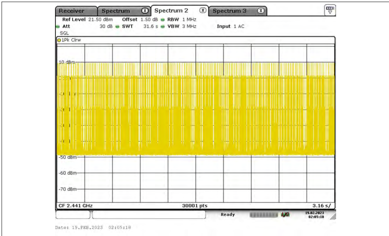
DH1_Ant1_Hop
