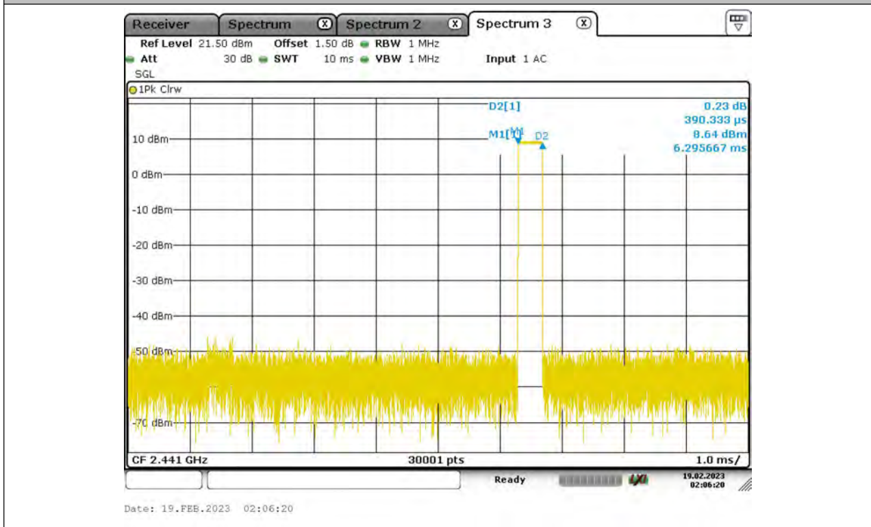
DH1_Ant1_Hop
