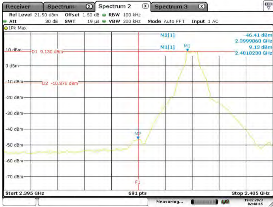
DH5_Ant1_Low_2402
