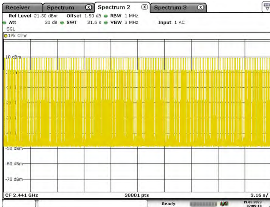
DH1_Ant1_Hop
