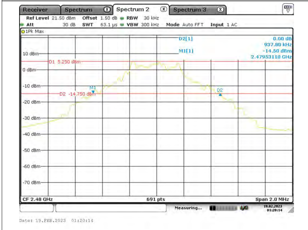
DH5_Ant1_2480
