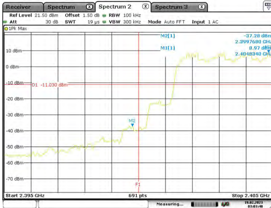
3DH5_Ant1_Low_Hop_2402
