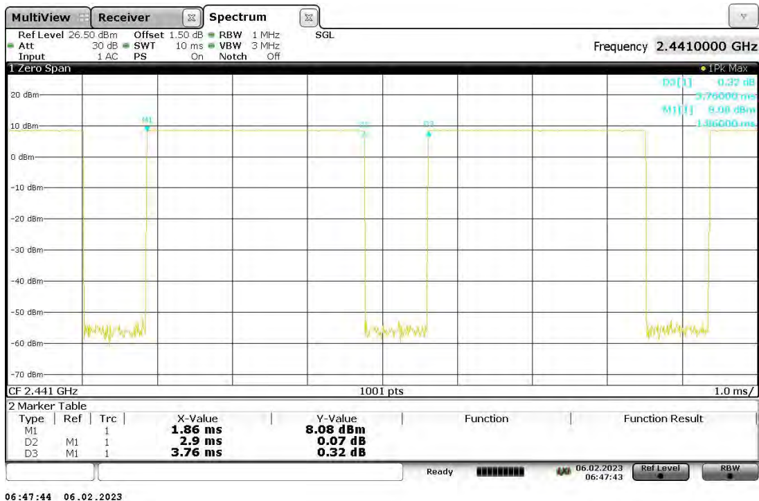
DH5_Ant1_2441
