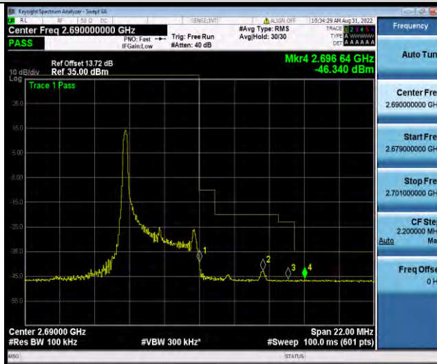
Band41-5MHz-16QAM-41565-1RB#24
