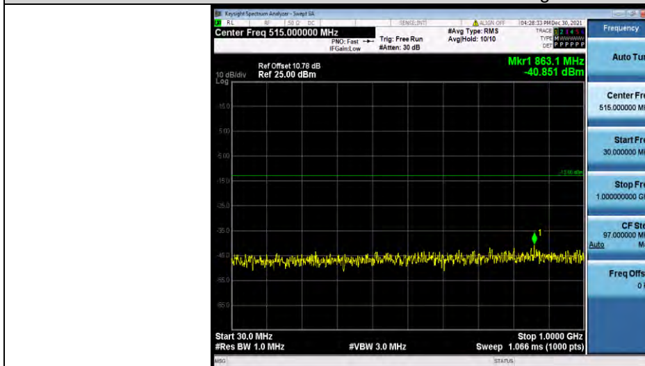
Band66-20MHz-QPSK-132572-1RB#0-Range2:1000~20000MHz
