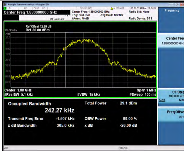
EGPRS1900-810-2-0.3086
