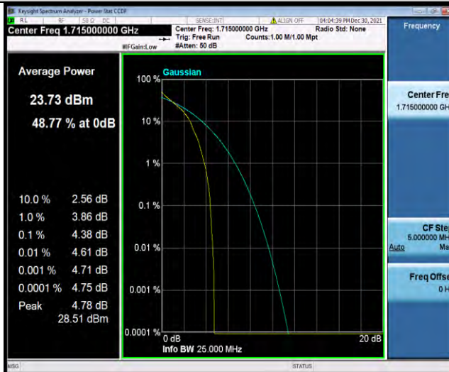
Band66-10MHz-QPSK-132022-50RB#0
