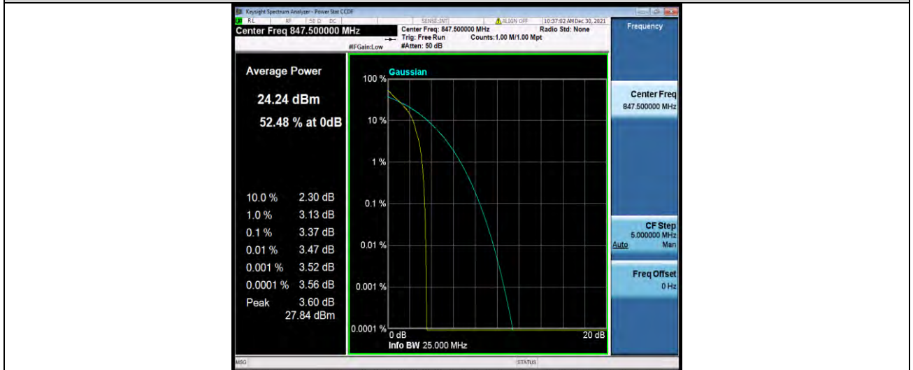
Band5-3MHz-QPSK-20635-15RB#0
