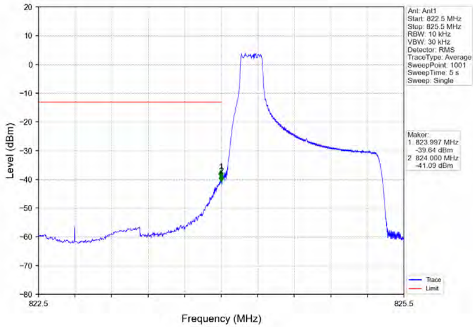
Band5 1.4MHz 64QAM LCH 824.7MHz RB 1 0 NTV
