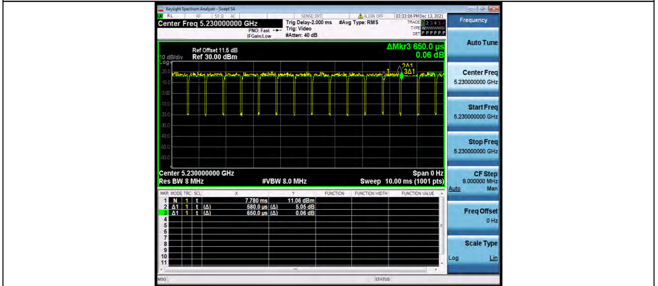
11N40SISO_Ant1_5230
