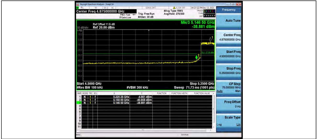
11AC80SISO_Ant1_Low_5210
