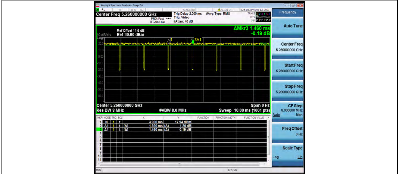
11A_Ant1_5260
