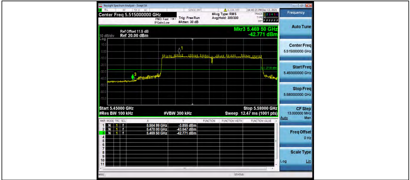
11AC80SISO_Ant1_Low_5530
