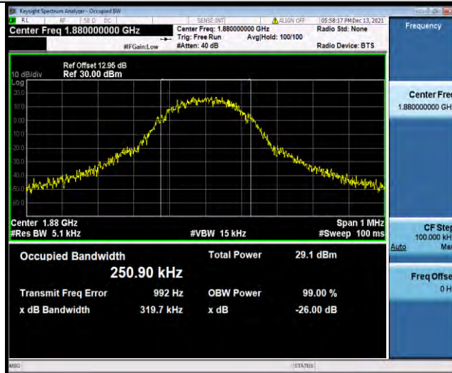
EGPRS1900-810-2-0.3103
