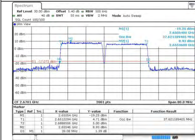
41-41-20MHz-20MHz-QPSK-QPSK-41292-41490-100 RB#0-100RB#0
