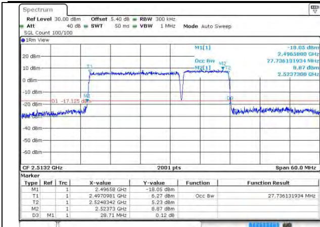
41-41-20MHz-10MHz-QPSK-QPSK-39750-39894-100 RB#0-50RB#0
