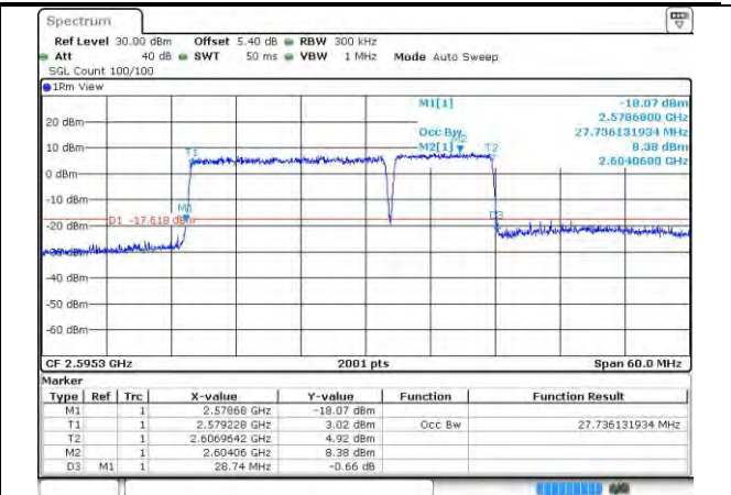
41-41-20MHz-10MHz-QPSK-QPSK-40571-40715-100 RB#0-50RB#0
