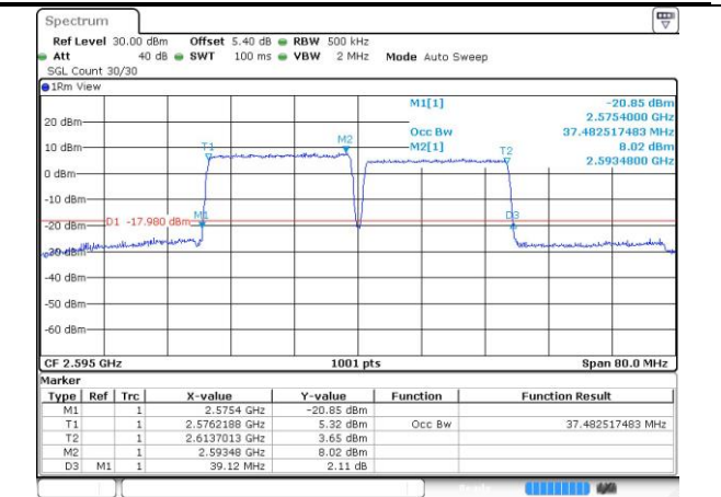
38-38-20MHz-20MHz-QPSK-QPSK-37901-38099-100 RB#0-100RB#0
