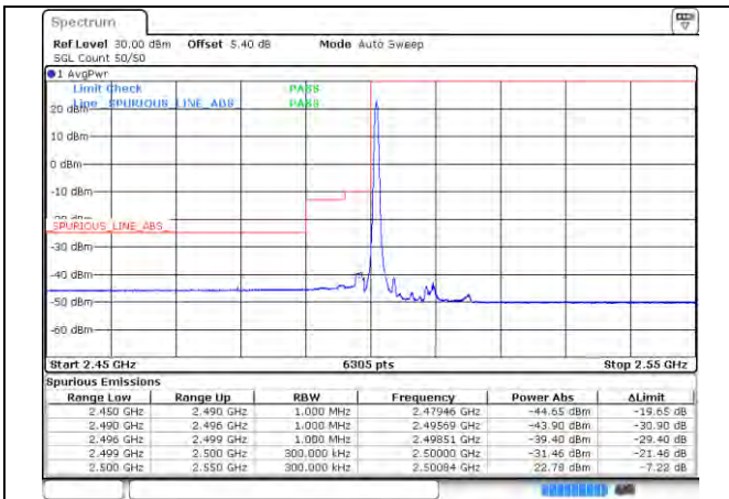
CA_7C_75RB+75RB_QPSK_20825+20975_1RB#0 +0RB#0
