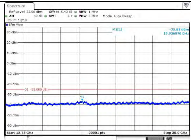
7-7-20MHz-20MHz-QPSK-QPSK-21001-21199 -ORB#0-1RB#99-12750~30000MHz
