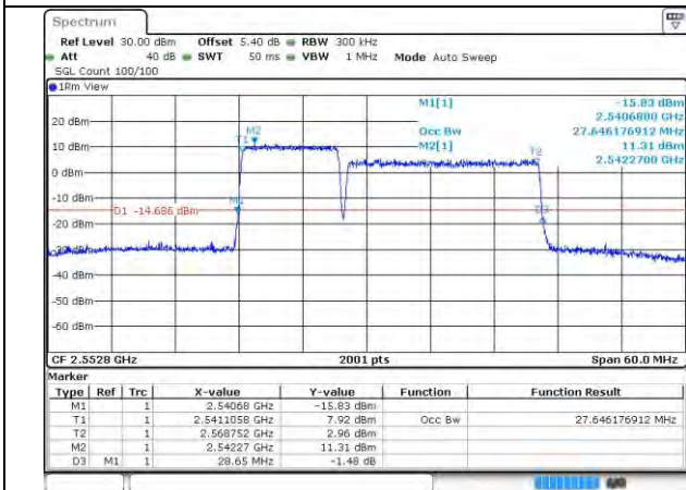
7-7-10MHz-20MHz-QPSK-QPSK-20805-20949-50RB #0-100RB#0
