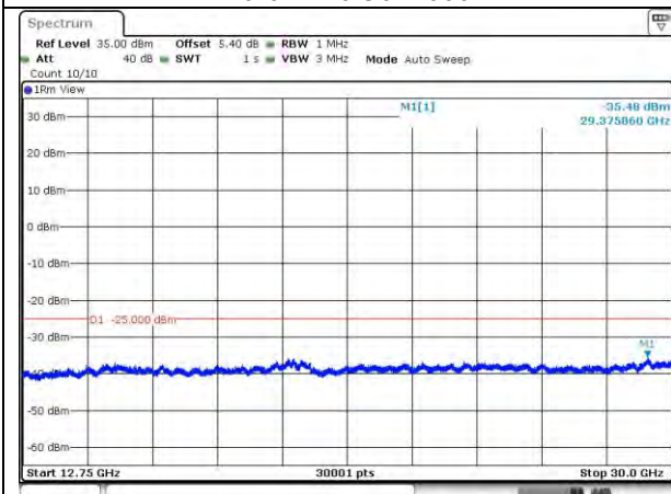
7-7-20MHz-20MHz-QPSK-QPSK-20850-21048 -1RB#0-ORB#0-12750~30000MHz
