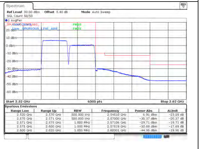
CA_7C_75RB+75RB_QPSK_21225+21375_75RB#0 +75RB#0
