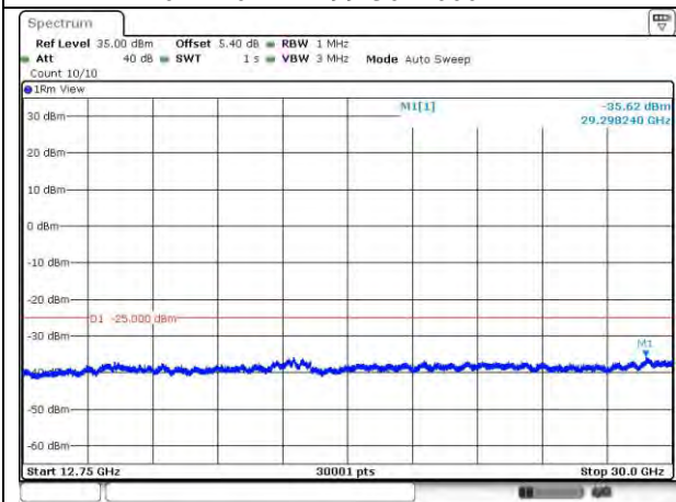
7-7-20MHz-20MHz-QPSK-QPSK-21152-21350 -ORB#0-1RB#99-12750~30000MHz
