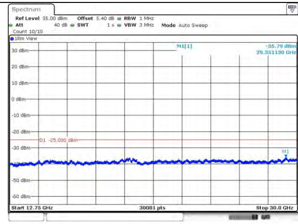
7-7-20MHz-20MHz-QPSK-QPSK-21001-21199 -1RB#0-0RB#0-12750~30000MHz
