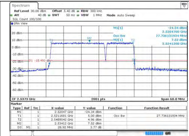
7-7-20MHz-10MHz-QPSK-QPSK-21051-21195-100RB #0-50RB#0
