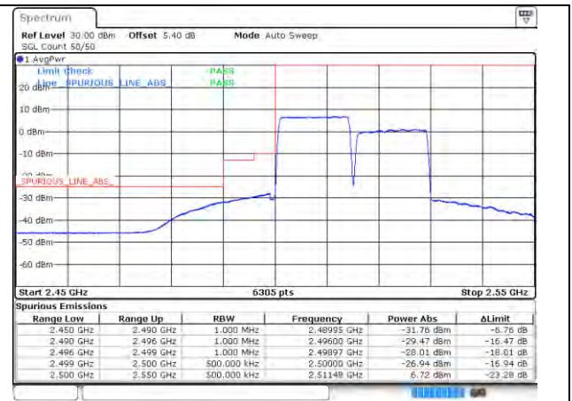
CA_7C_75RB+75RB_QPSK_20825+20975_75RB#0 +75RB#0
