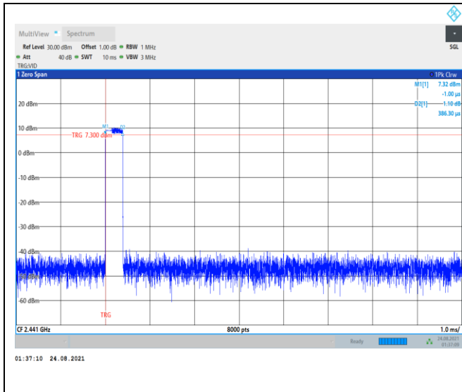
Modulation: \pi/4 DQPSK DH1 2441
