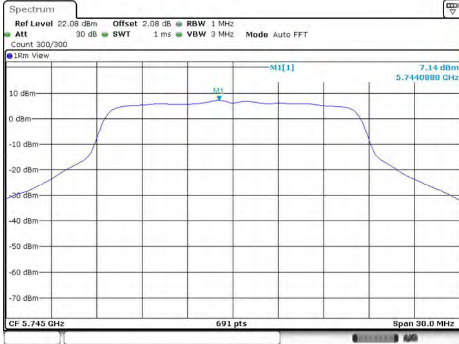
11A_Ant10_5745
