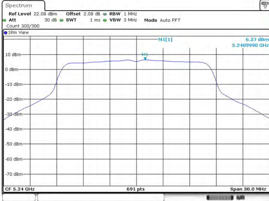
11A_Ant10_5240
