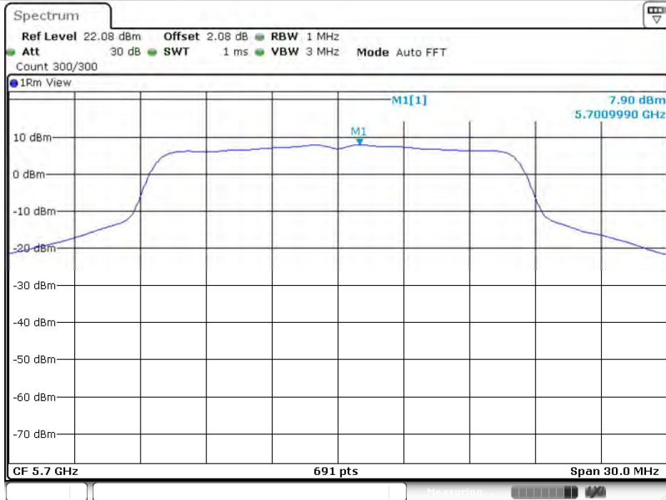
11A_Ant9_5700
