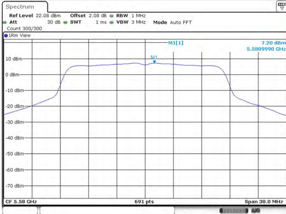
11A_Ant9_5580
