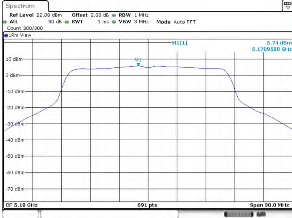
11A_Ant10_5180
