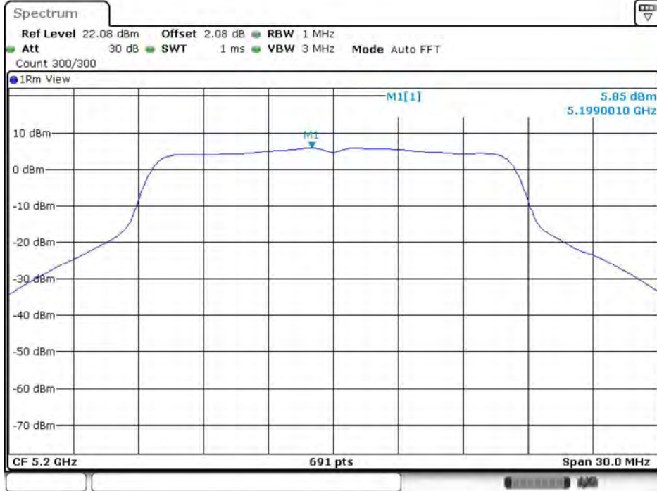
11A_Ant10_5200
