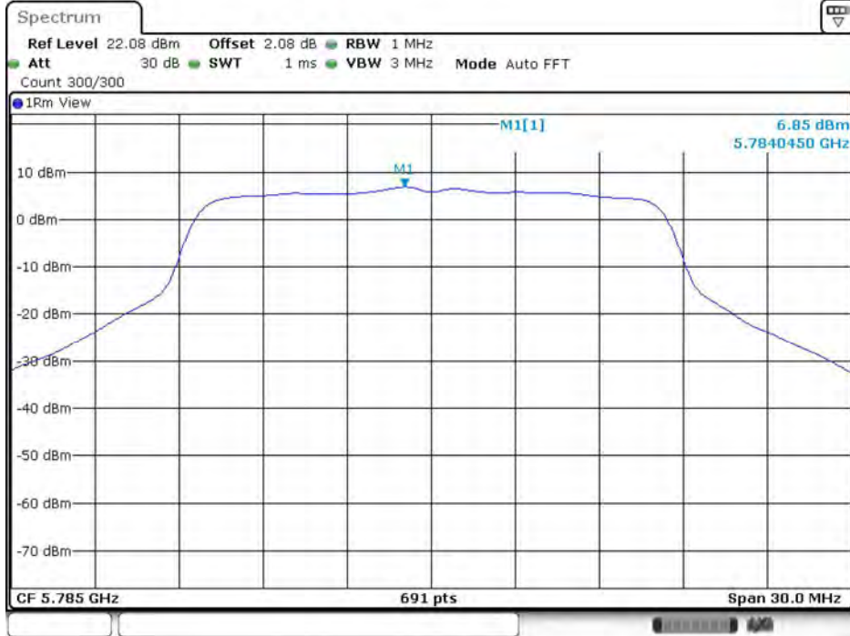
11A_Ant10_5785
