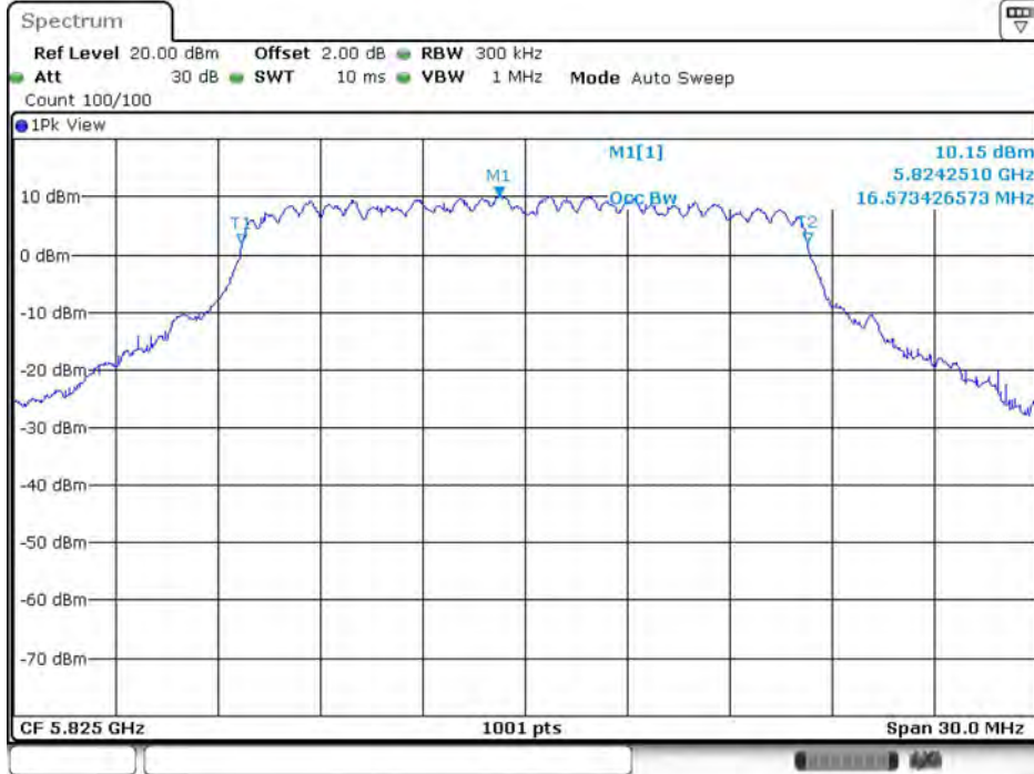
11A-CDD_Ant10_5825
