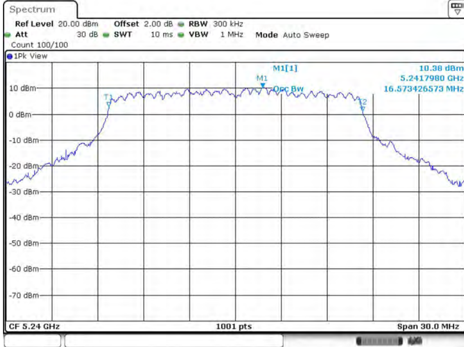
11A-CDD_Ant10_5240
