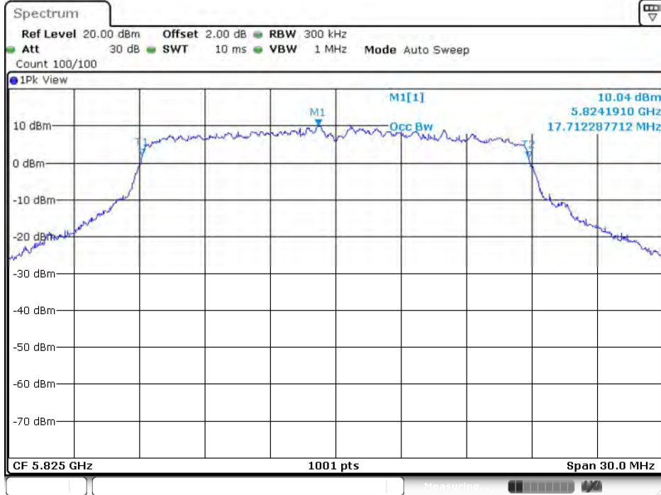
11N20SISO_Ant10_5825
