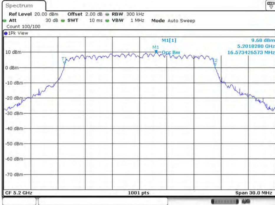
11A-CDD_Ant10_5200
