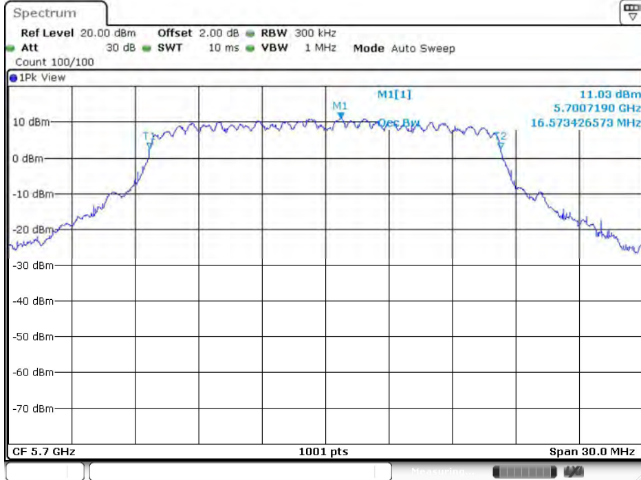
11A-CDD_Ant10_5700
