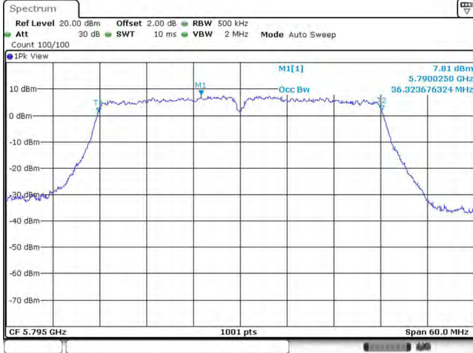
11N40SISO_Ant10_5795
