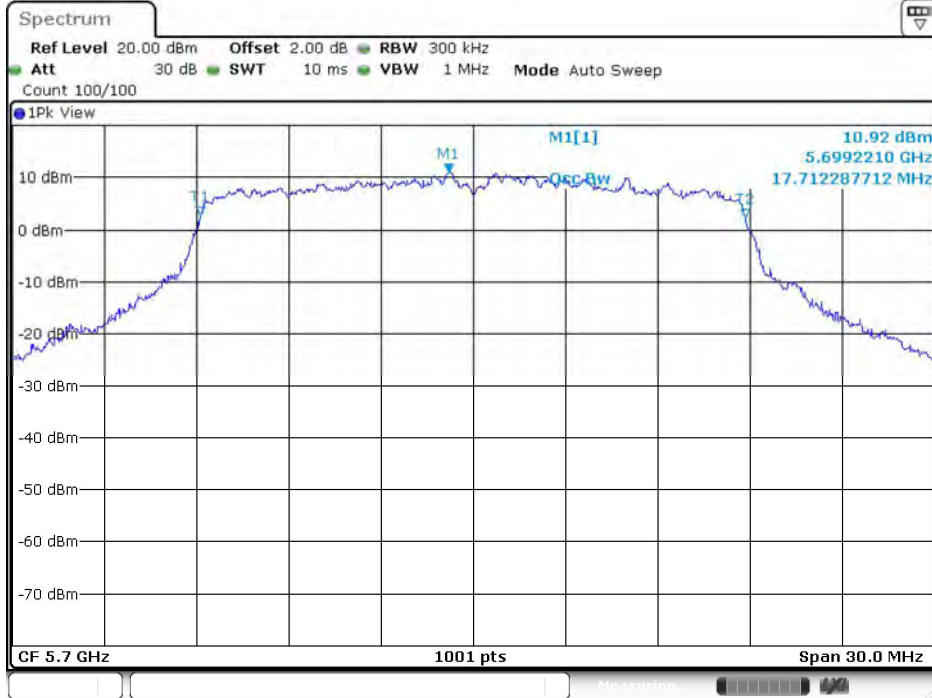
11N20MIMO_Ant10_5700
