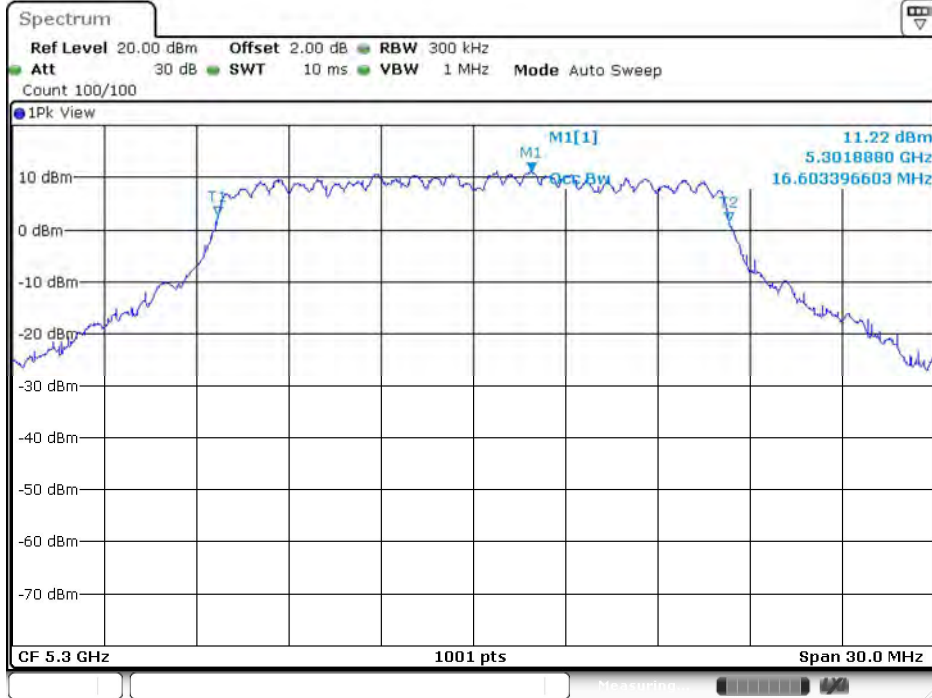
11A-CDD_Ant10_5300
