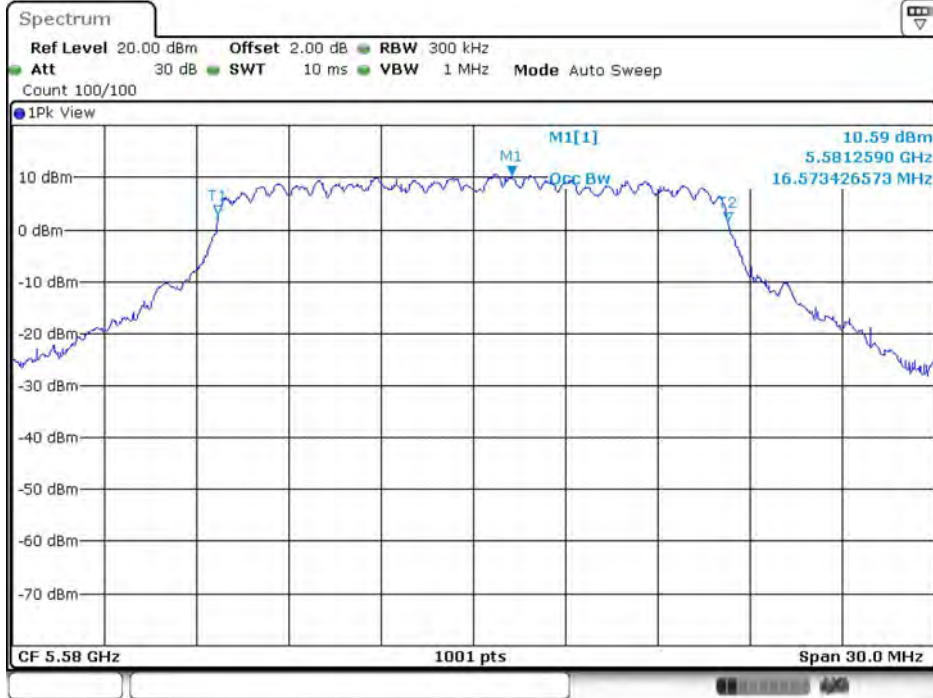
11A-CDD_Ant10_5580
