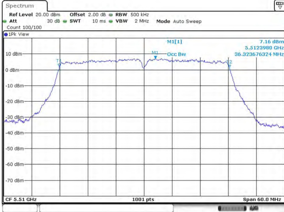
11N40SISO_Ant10_5510
