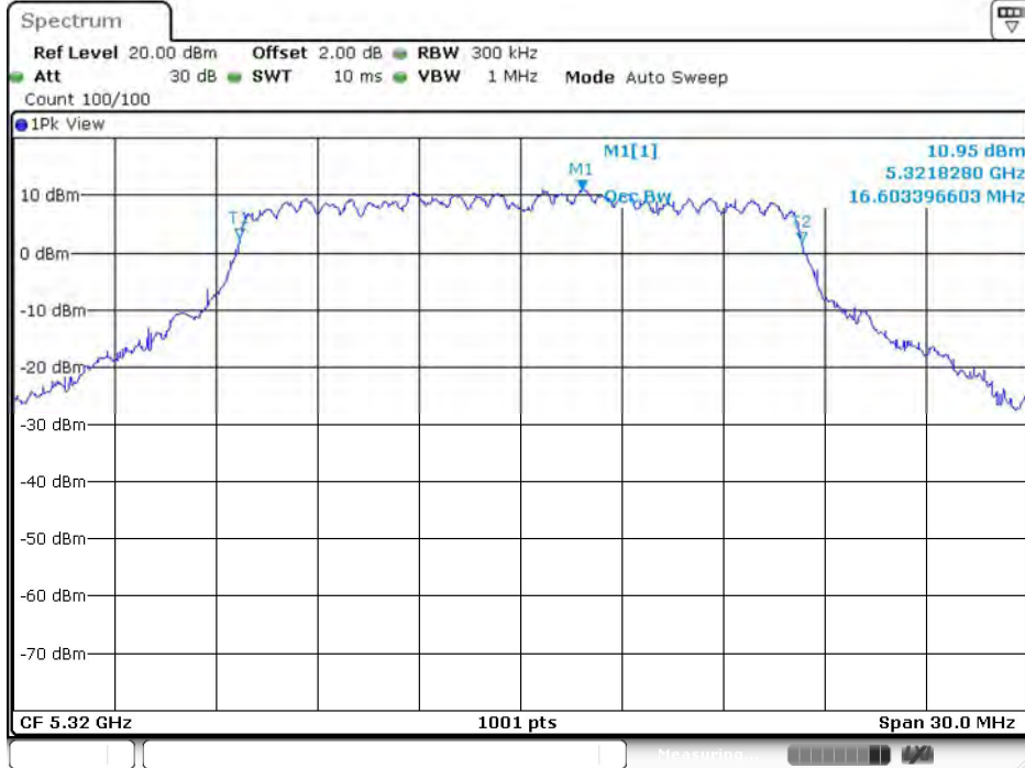
11A-CDD_Ant10_5320
