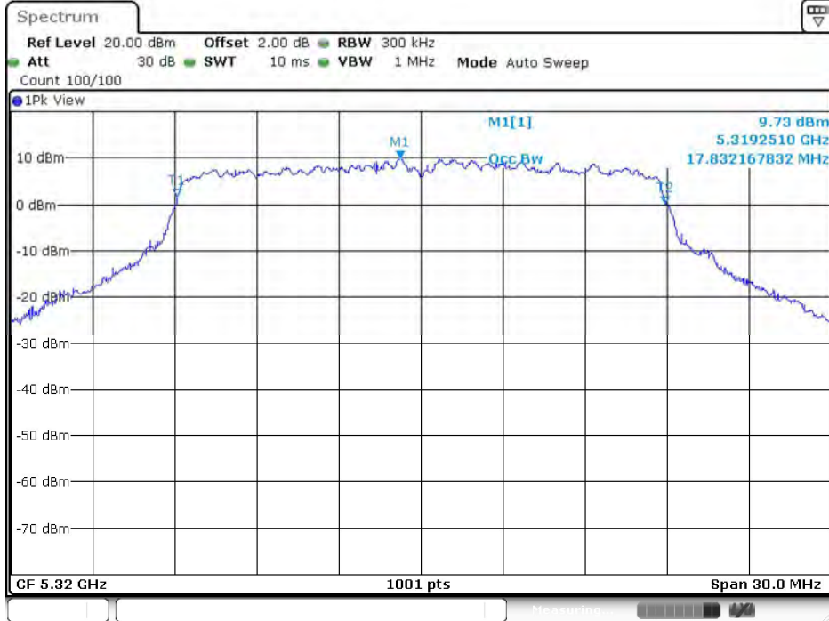
11N20SISO_Ant10_5320
