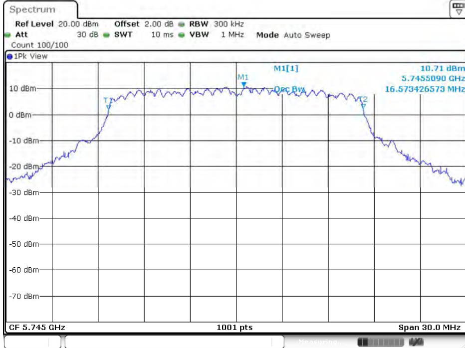
11A-CDD_Ant10_5745
