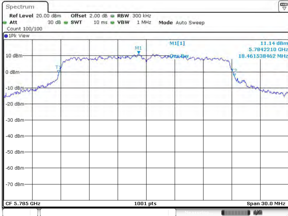
11N20MIMO_Ant9_5785
