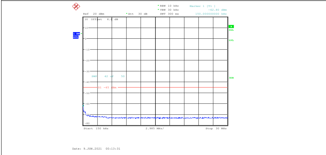
NTNV-DC_2A_n41A-30kHz-5MHz+100MHz-N/A+DFT-PI2BPSK-Mid+Low-N/A-Edge_1RB_L eft-0.15-30-----45-PASS
