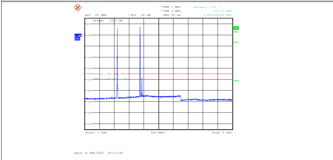
NTNV-DC_2A_n41A-30kHz-5MHz+100MHz-N/A+DFT-PI2BPSK-Mid+Low-N/A-Edge_1RB_L eft-1000-5000-----25-PASS
