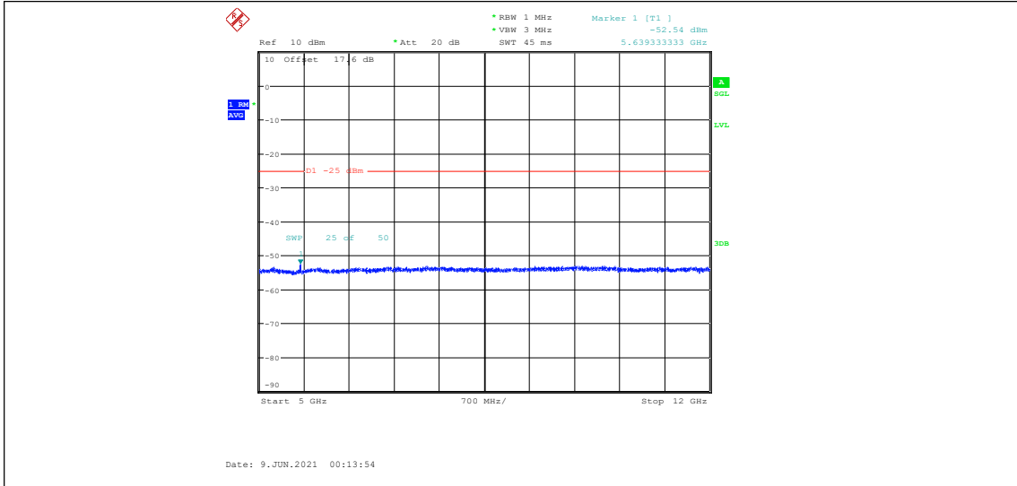
NTNV-DC_2A_n41A-30kHz-5MHz+100MHz-N/A+DFT-PI2BPSK-Mid+Low-N/A-Edge_1RB_L eft-5000-12000-----25-PASS
