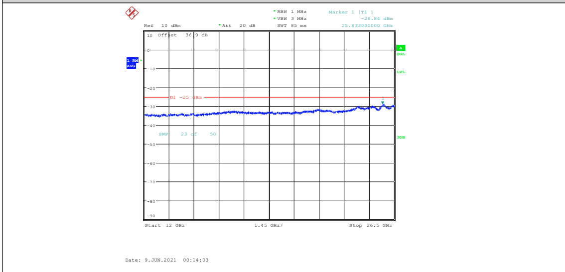
NTNV-DC_2A_n41A-30kHz-5MHz+100MHz-N/A+DFT-PI2BPSK-Mid+Low-N/A-Edge_1RB_L eft-12000-26500-----25-PASS
