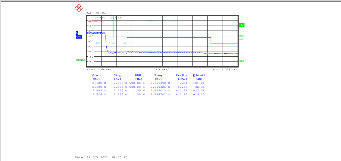
NTNV-DC_2A_n41A-30kHz-5MHz+40MHz-N/A+DFT-PI2BPSK-Mid+High-N/A-Outer_Full----- -----see graph-PASS
