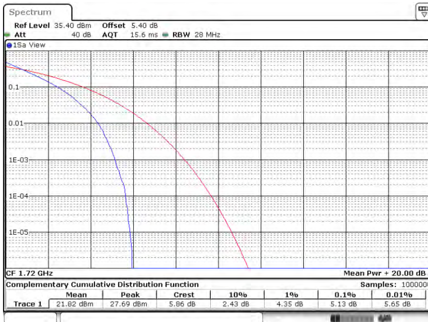
Band4-20MHz-QPSK-20050-100RB#0
