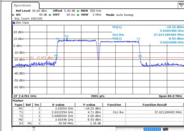
41-41-20MHz-20MHz-QPSK-QPSK-41292-41490-100 RB#0-100RB#0
