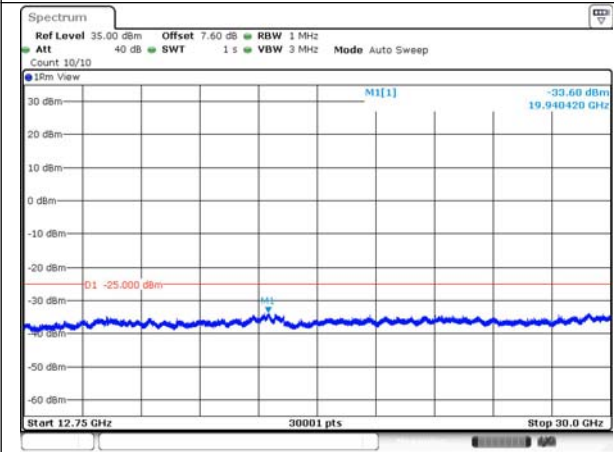
41-41-20MHz-20MHz-QPSK-QPSK-41292-41490 -1RB#0-ORB#0-12750~30000MHz
