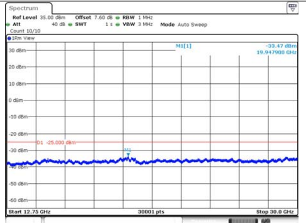
41-41-20MHz-20MHz-QPSK-QPSK-40521-40719 -1RB#0-0RB#0-12750~30000MHz
