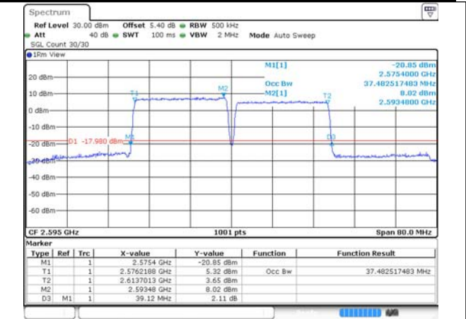
38-38-20MHz-20MHz-QPSK-QPSK-37901-38099-100 RB#0-100RB#0
