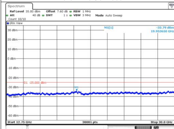
38-38-20MHz-20MHz-QPSK-QPSK-37952-38150 -1RB#0-ORB#0-12750~30000MHz
