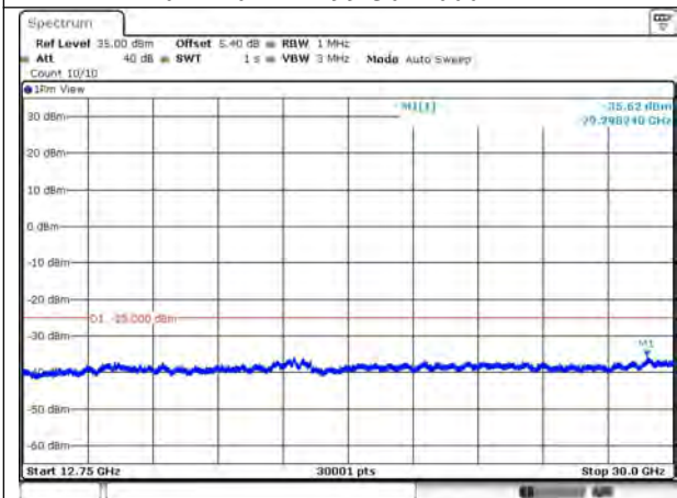
7-7-20MHz-20MHz-QPSK-QPSK-21152-21350 -ORB#0-1RB#99-12750~30000MHz
