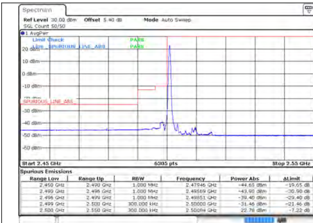
CA_7C_75RB+75RB_QPSK_20825+20975_1RB#0+0RB#0
