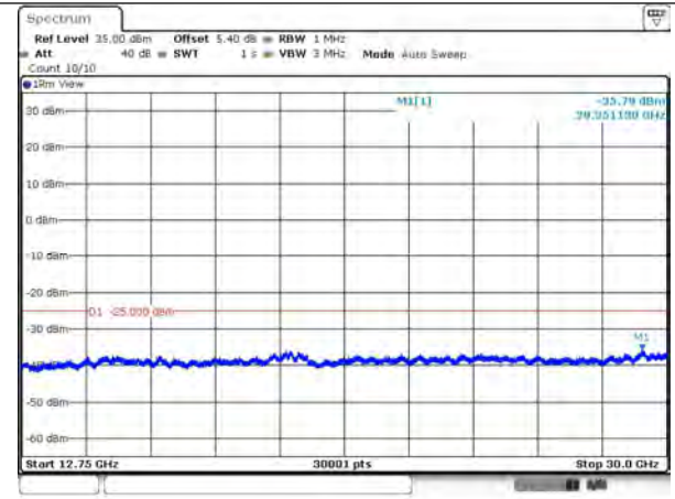
7-7-20MHz-20MHz-QPSK-QPSK-21001-21199 -1RB#0-0RB#0-12750~30000MHz
