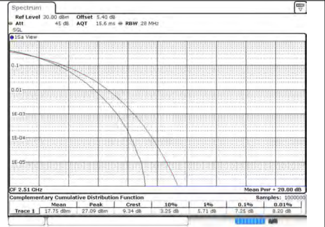
CA_7C_100RB+100RB_64QAM_21199+21001_100RB#0+100RB#0
