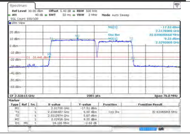
7-7-20MHz-15MHz-QPSK-QPSK-21026-21197-100RB #0-75RB#0
