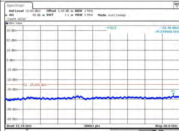
7-7-20MHz-20MHz-QPSK-QPSK-20850-21048 -1RB#0-ORB#0-12750~30000MHz
