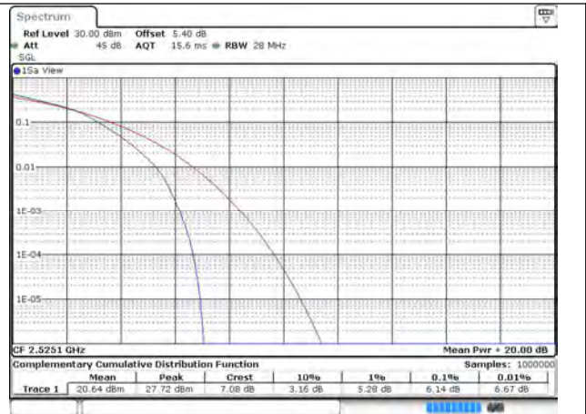
CA_7C_100RB+100RB_64QAM_21199+21001_100RB#0+100RB#0
