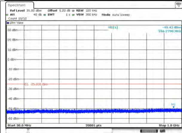
7-7-20MHz-20MHz-QPSK-QPSK-20850-21048 -1RB#0-ORB#0-30~1000MHz
