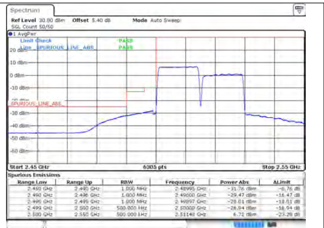
CA_7C_75RB+75RB_QPSK_20825+20975_75RB#0+75RB#0
