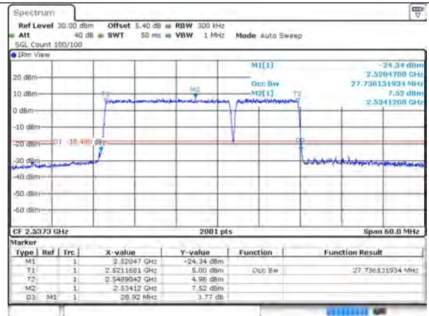
7-7-20MHz-10MHz-QPSK-QPSK-21051-21195-100RB #0-50RB#0
