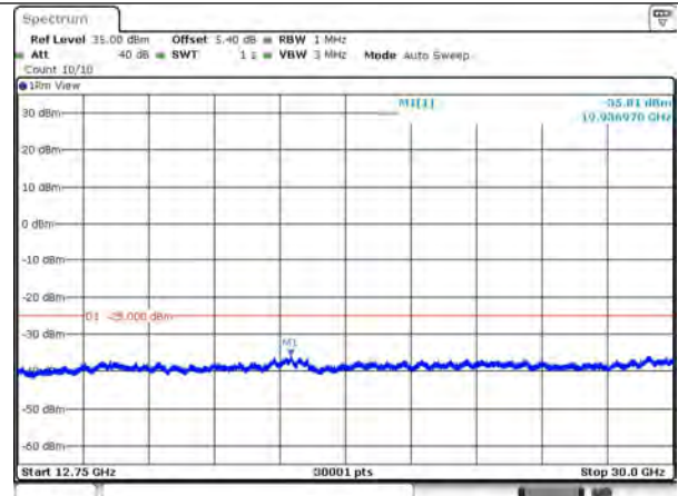
7-7-20MHz-20MHz-QPSK-QPSK-21001-21199 -ORB#0-1RB#99-12750~30000MHz
