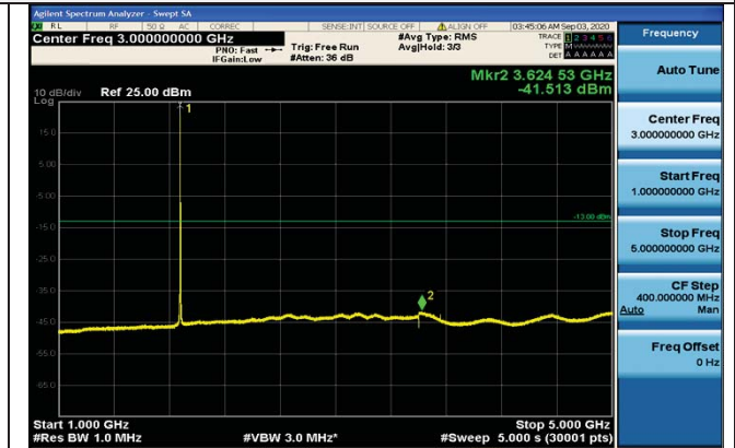
1GHz~5GHz
