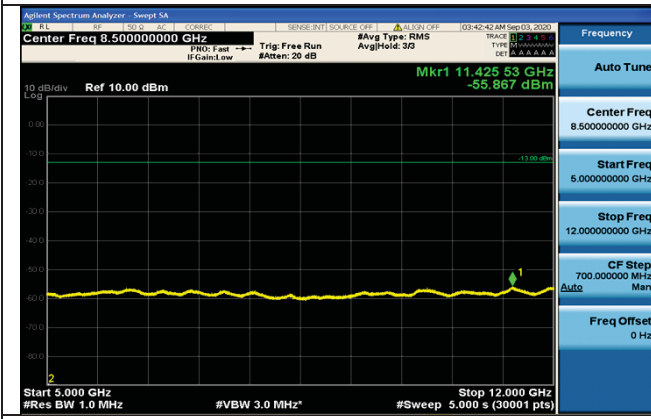
5GHz~12GHz
