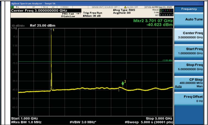
1GHz~5GHz
