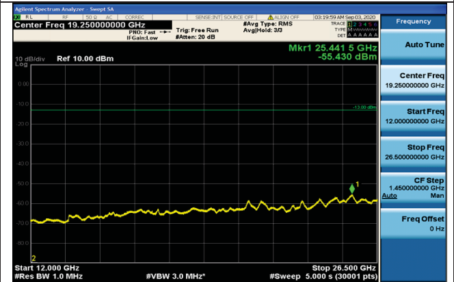
12GHz~26.5GHz
