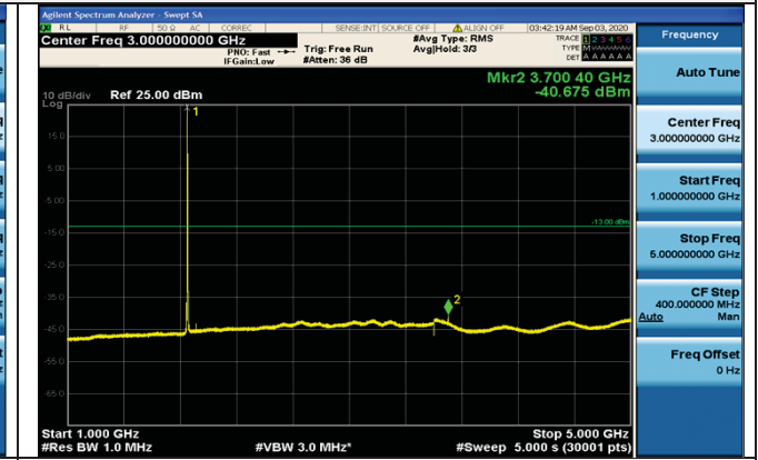
1GHz~5GHz
