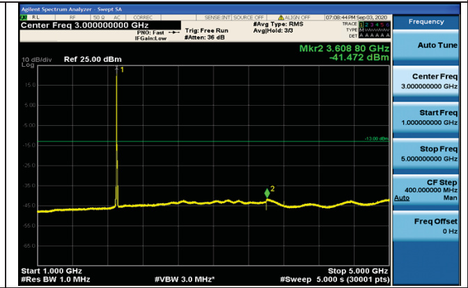
1GHz~5GHz
