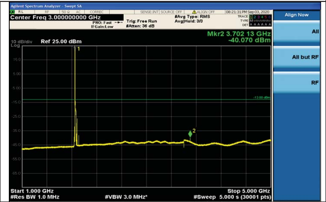
1GHz~5GHz
