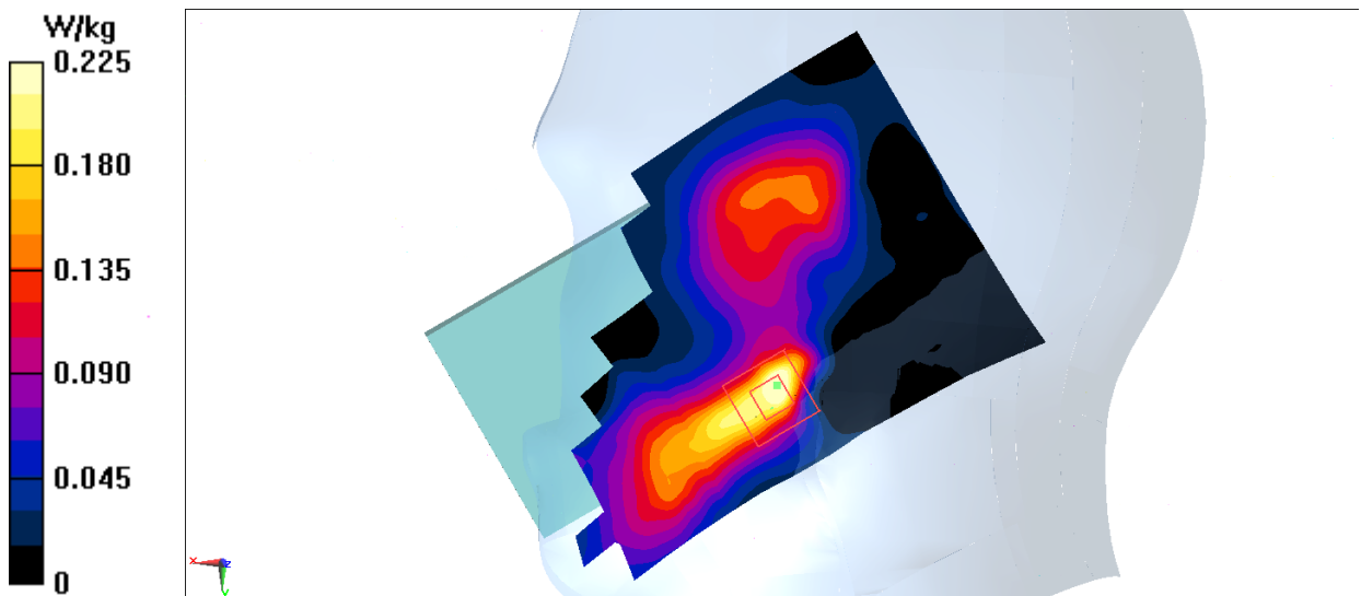
Fig.15 LTE Band7
