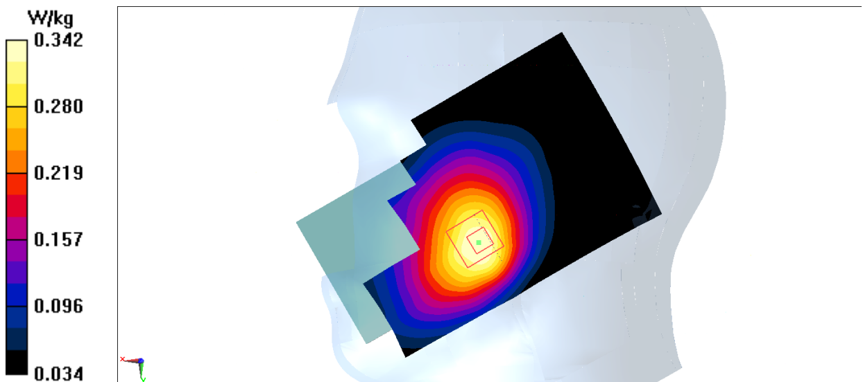
Fig.13 LTE Band5
