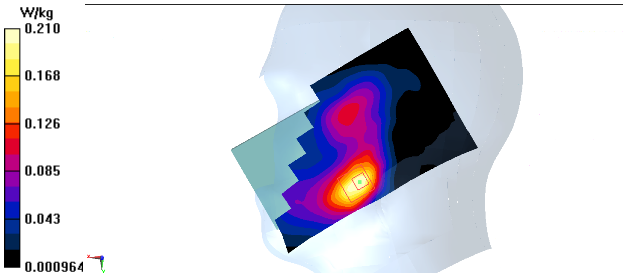
Fig.11 LTE Band2
