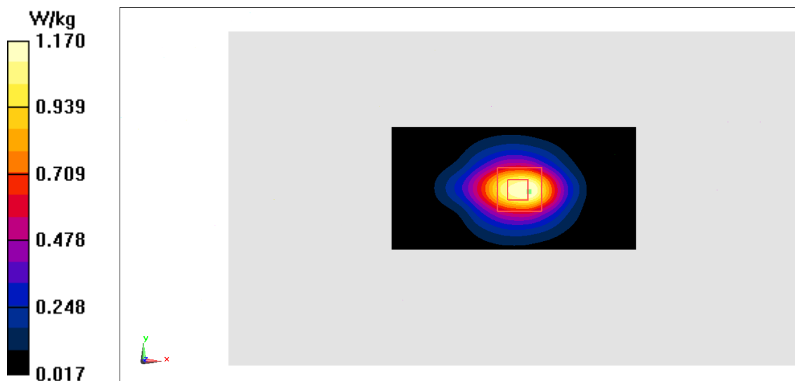
Fig.12 LTE Band2
