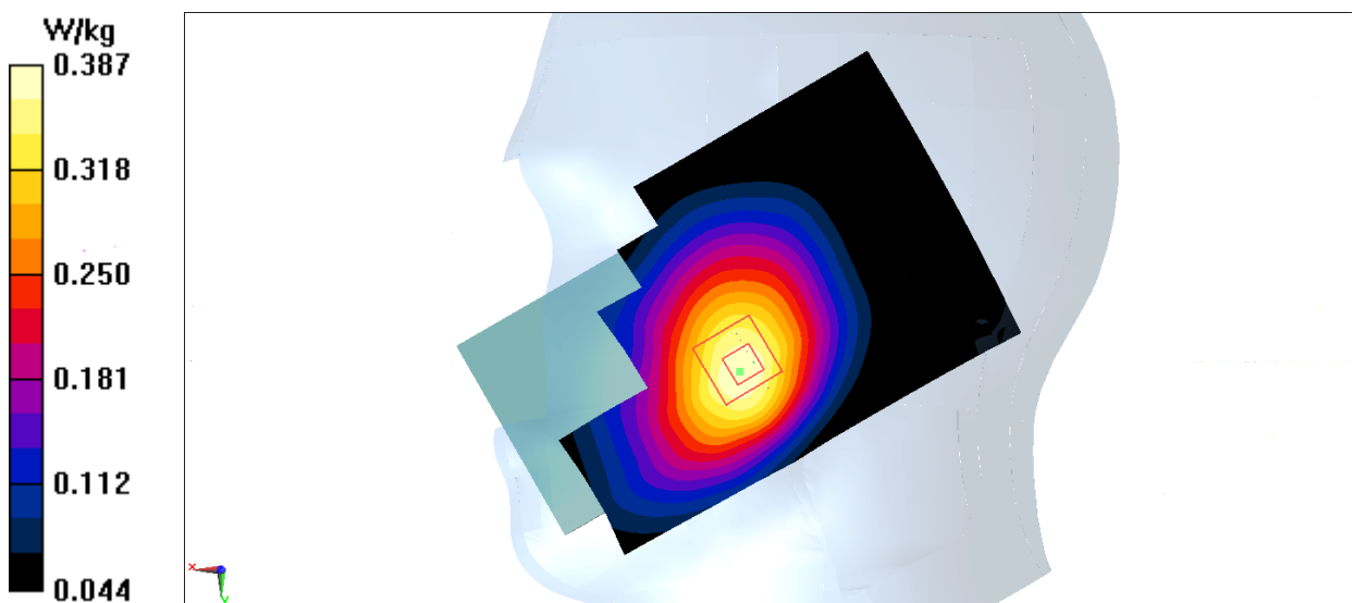
Fig.5 WCDMA 850
