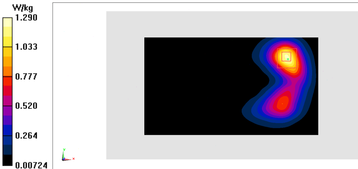
Fig.16 LTE Band7
