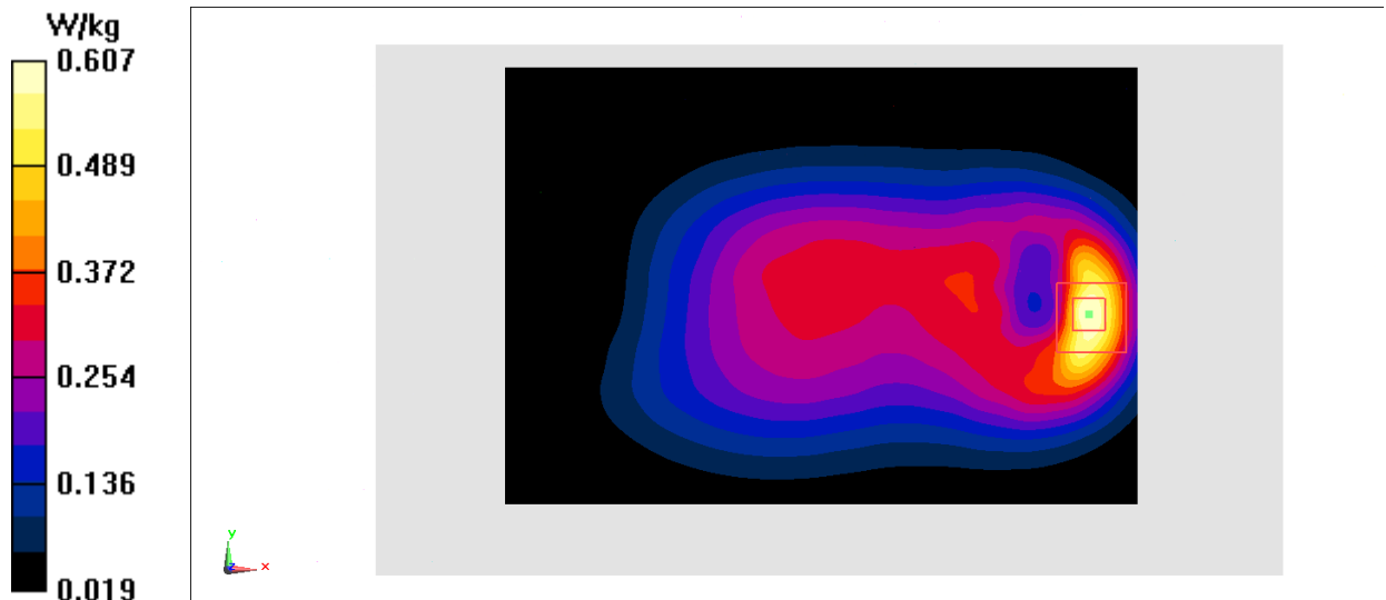
Fig.14 LTE Band5
