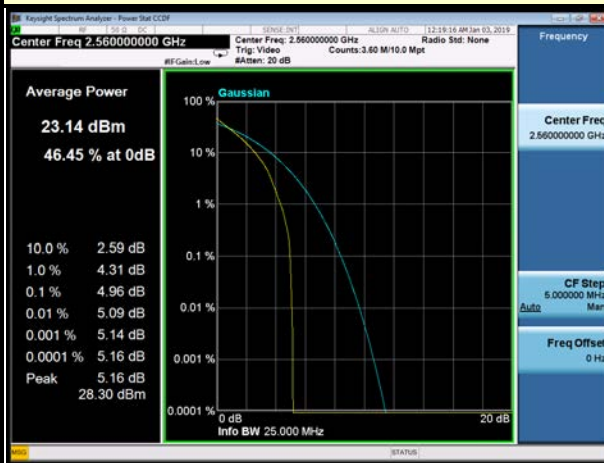
20MHz / QPSK
