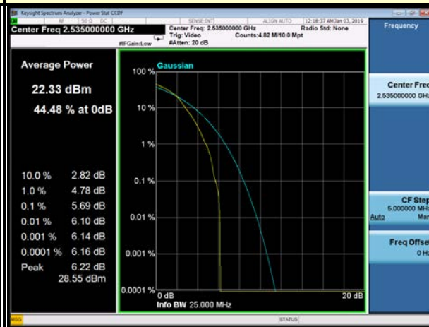
20MHz / 16QAM
