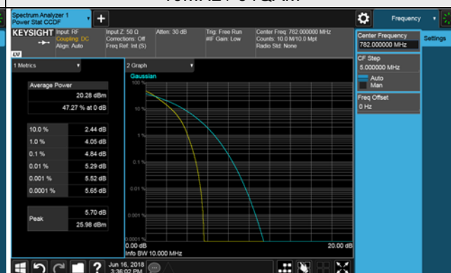
10MHz / 64QAM
