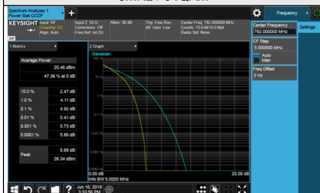
5MHz / 64QAM
