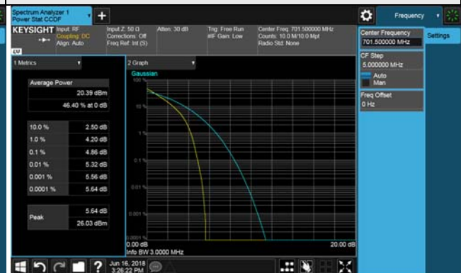
10MHz / 16QAM
