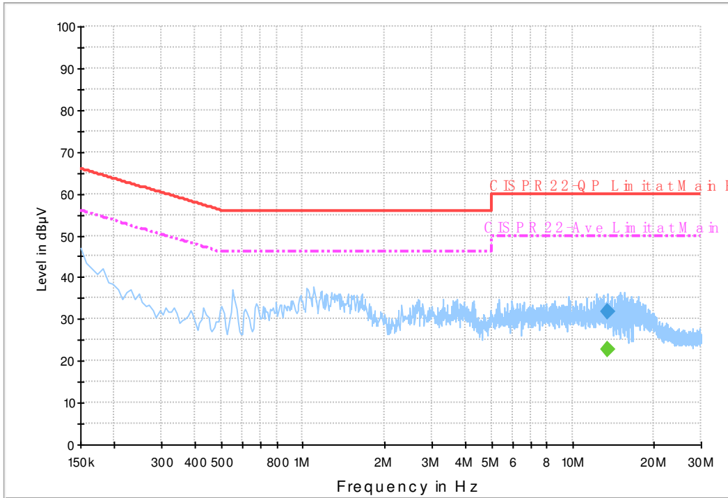
ENV216 Auto Test NCC CE Power Bar - L
