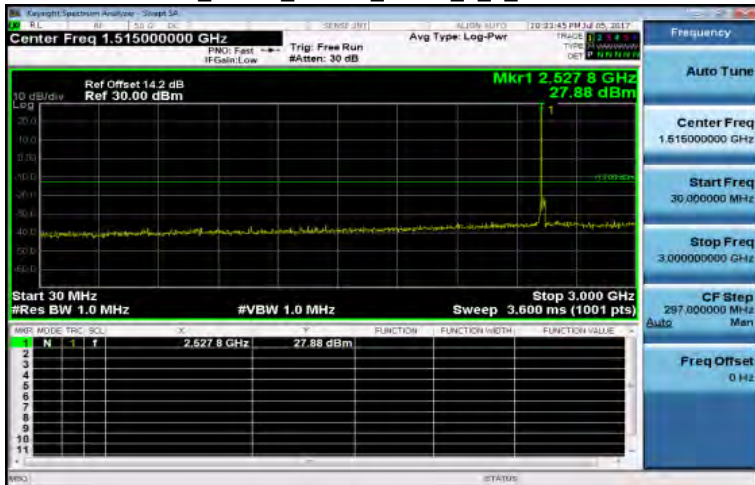
30MHz-3GHz_Band7_20MHz_QPSK_1_0_MidCH21100-2535
