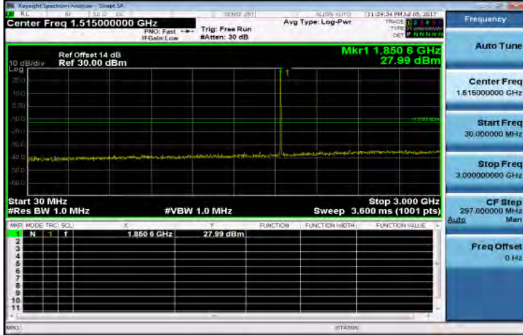
30MHz~3GHz_Band2_3MHz_QPSK_1_0_LowCH18615-1851.5
