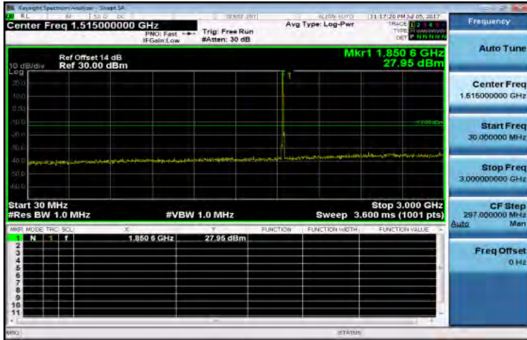
30MHz-3GHz_Band2_10MHz_QPSK_1_0_LowCH18650-1855
