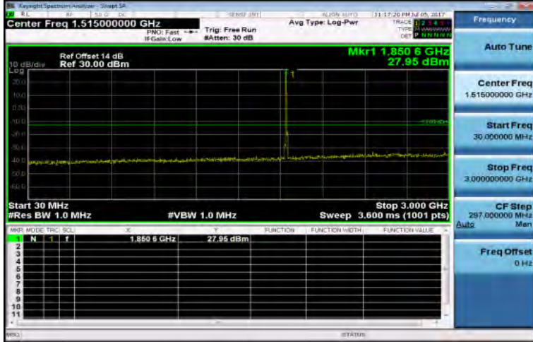
30MHz-3GHz_Band2_10MHz_QPSK_1_0_LowCH18650-1855
