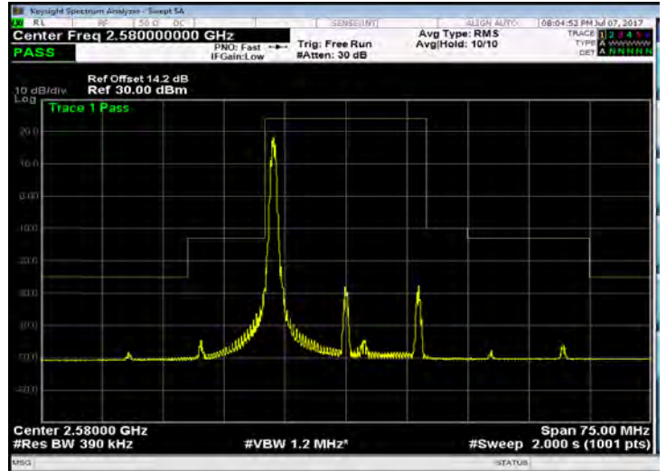
Band 38_20M_16QAM_LOW_RB1,99
