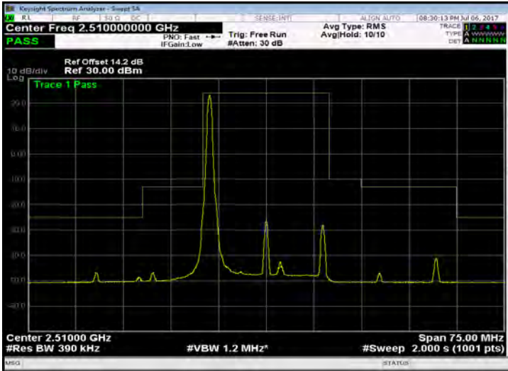
Band 7_20M_QPSK_LOW_RB1,99
