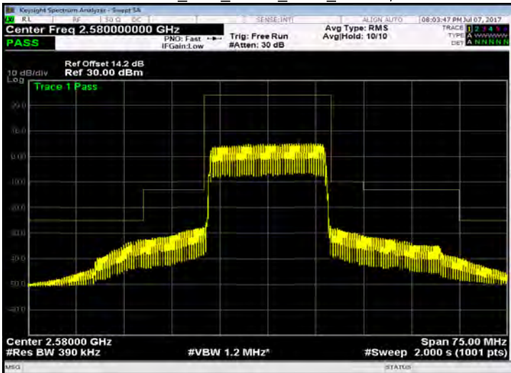
Band 38_20M_QPSK_LOW_RB100,0
