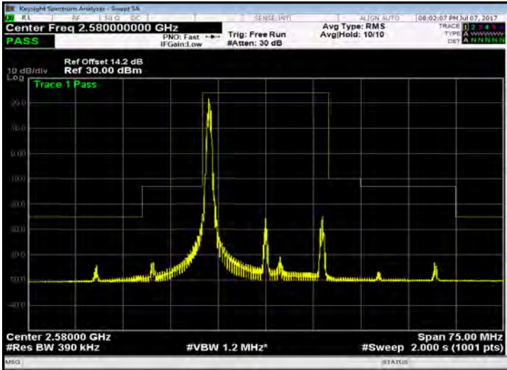
Band 38_20M_QPSK_LOW_RB1,99
