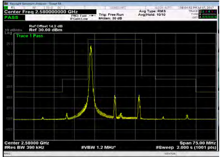
Band 38_20M_16QAM_LOW_RB1,99
