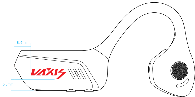
logo丝印白色, 尺寸18*5.6mm
