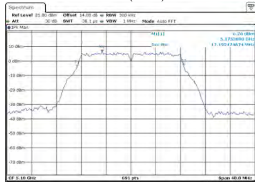
ANT 2(11A)
