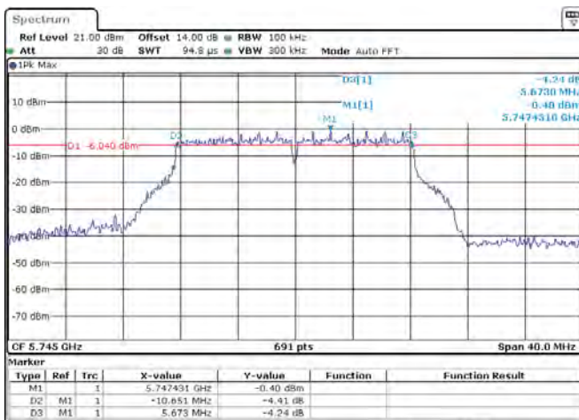
ANT 1(802.11A)
