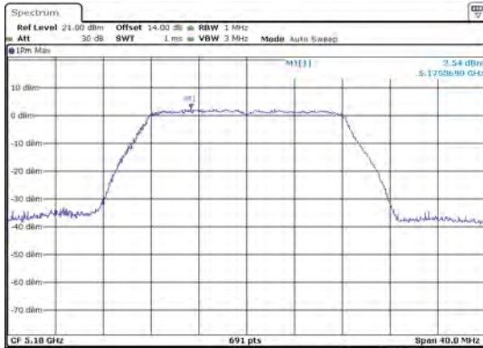
ANT 1(11A)
