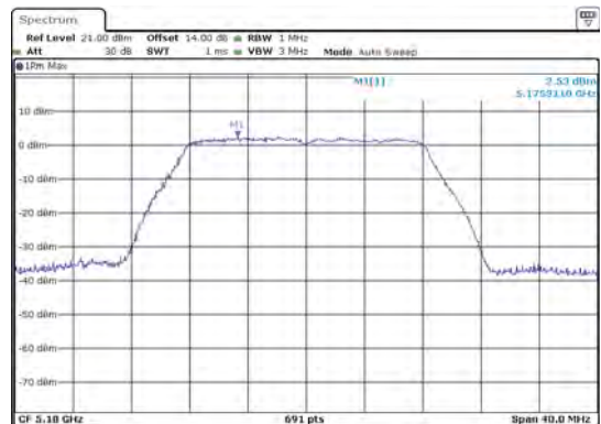
ANT 2(11A)
