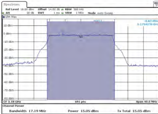
ANT 1(802.11A)
