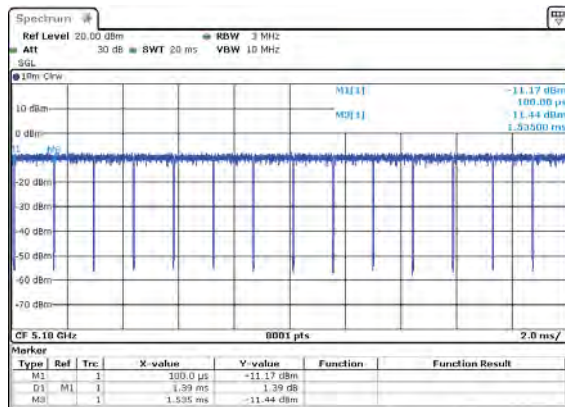
ANT 1
