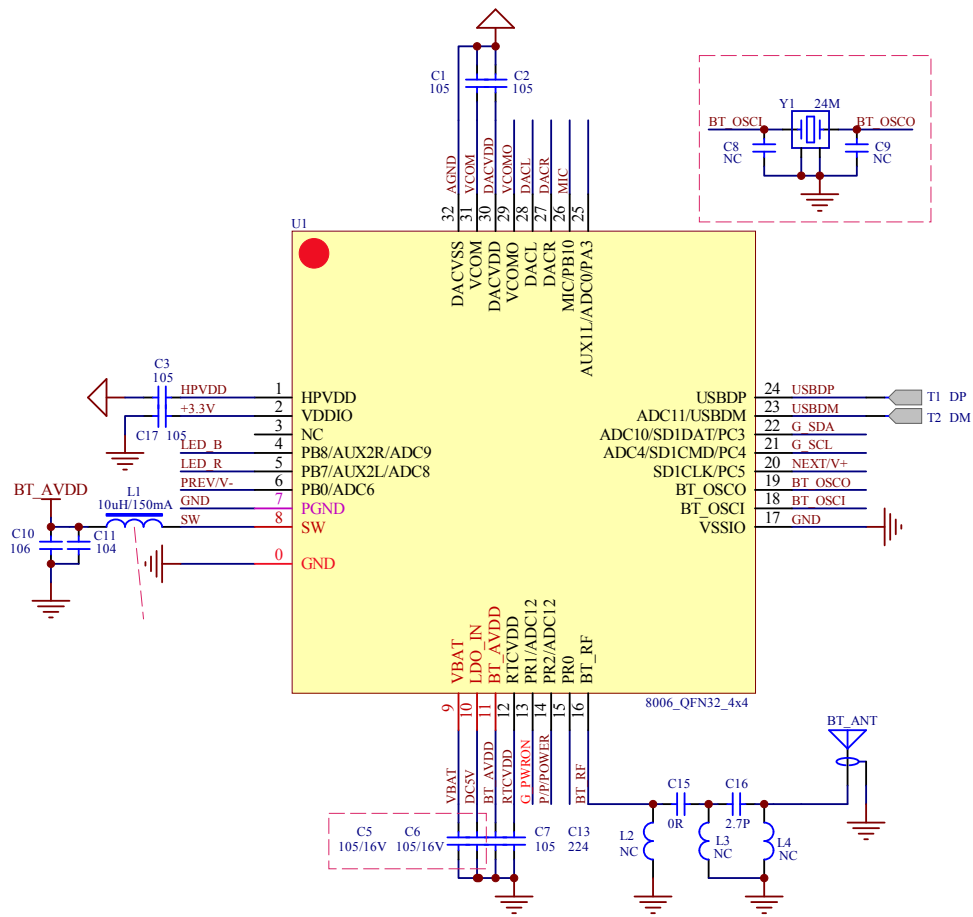
MCU
