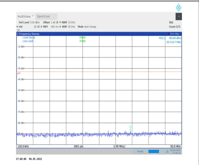
1-N78-3700-3800--30-100-M-1-DFT-PI2BPSK- Inner_1RB_Left-1@1-0.15-30-Ant0--86.88--33-PASS
