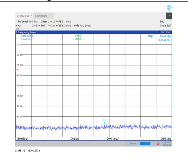
1-N78-3700-3800--30-100-H-1-DFT-PI2BPSK- Inner_1RB_Left-1@1-0.15-30-Ant0--86.69--33-PASS
