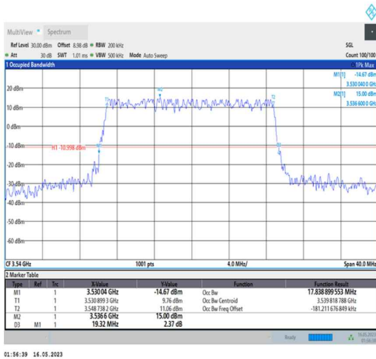
1-N78-3450-3550-PC1-30-20-H-3-DFT-16QAM-Outer_Full-50@0-Ant0-17.839-19.320-≤20-PASS
