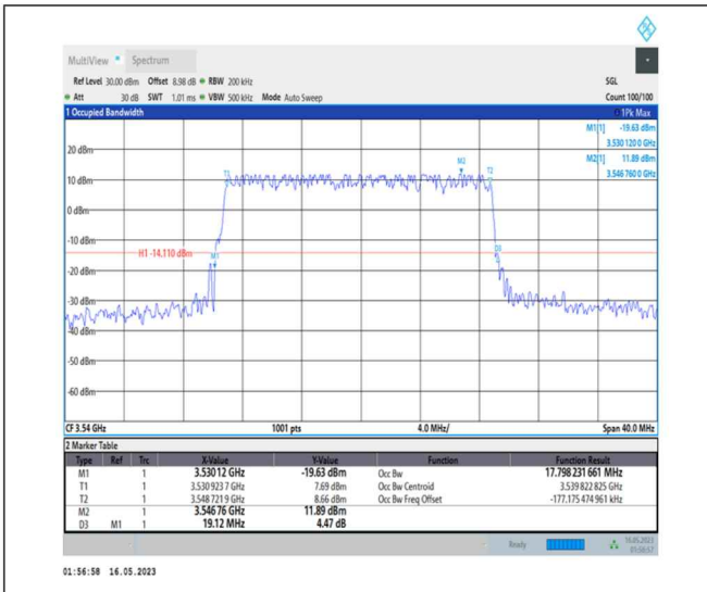
1-N78-3450-3550-PC1-30-20-H-5-DFT-256QAM-Outer_Full-50@0-Ant0-17.798-19.120-≤20-PASS
