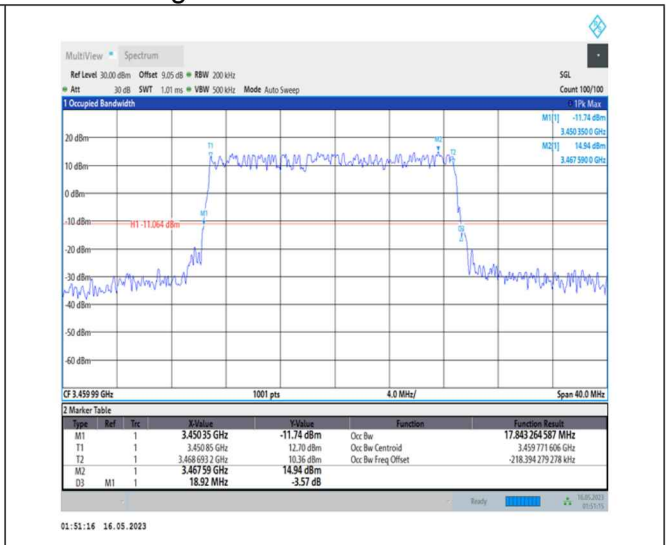
1-N78-3450-3550-PC1-30-20-L-4-DFT-64QAM-Outer_Full-50@0-Ant0-17.843-18.920-≤20-PASS
