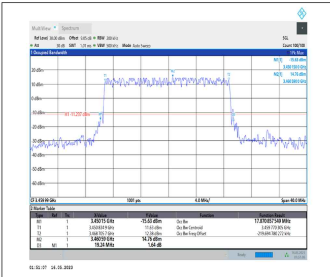
1-N78-3450-3550-PC1-30-20-L-3-DFT-16QAM-Outer_Full-50@0-Ant0-17.871-19.240-≤20-PASS
