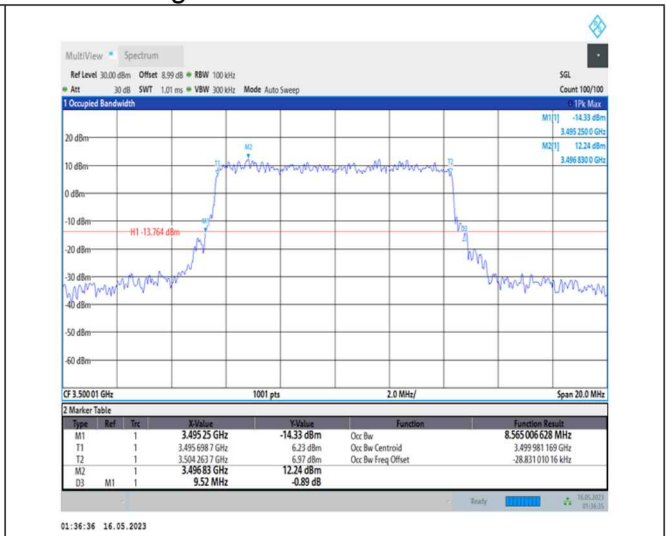
1-N78-3450-3550-PC1-30-10-M-5-DFT-256QAM-Outer_Full-24@0-Ant0-8.565-9.520-≤10-PASS
