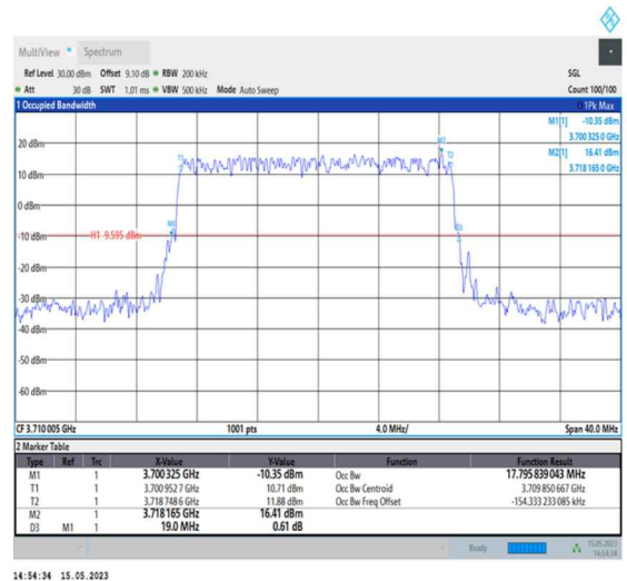
1-N77-3700-3980-PC1-30-20-L-2-DFT-PI2BPSK-Outer_Full-50@0-Ant0-17.796-19.000-≤20-PASS
