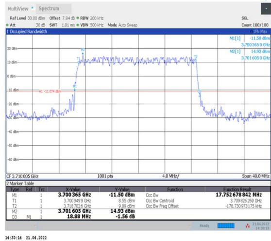
1-N77-3700-3980--30-20-L-2-DFT-P12BPSK-Outer_Full-50@0-Ant0-17.753-18.880-≤20-PASS
