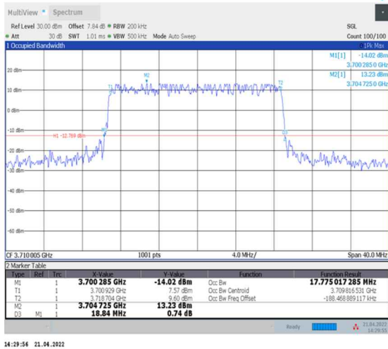
1-N77-3700-3980--30-20-L-1-DFT-QPSK-Outer_Full-50@0-Ant0-17.775-18.840-≤20-PASS
