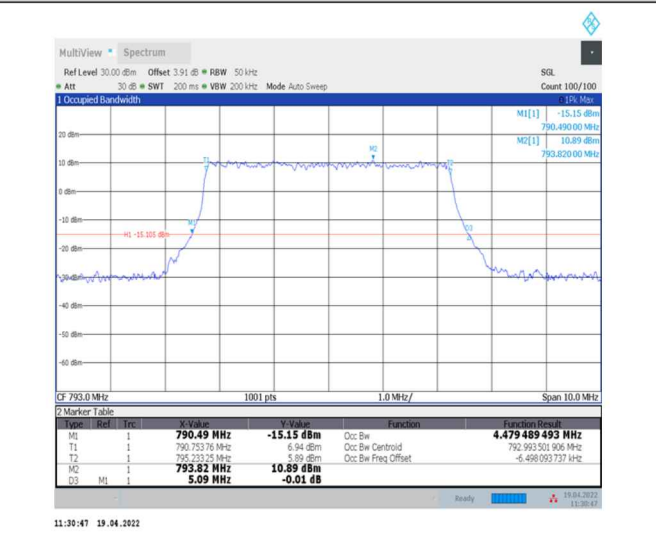
1-N14--15-5-M-7-CP-16QAM-Outer_Full-25@0-Ant0-4.479-5.090-≤5-PASS
