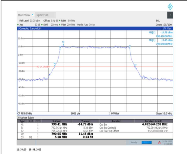
1-N14--15-5-M-6-CP-QPSK-Outer_Full-25@0-Ant0-4.483-5.180-≤5-PASS
