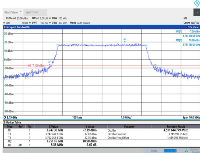
Band43-5MHz-QPSK-45090-25RB#0
