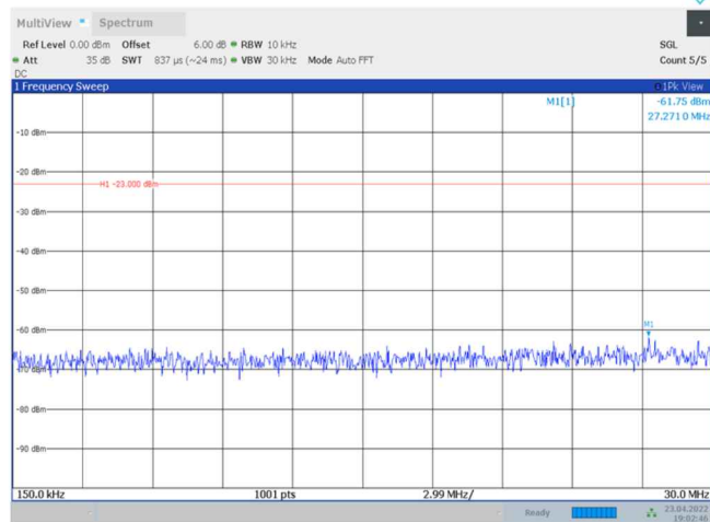
Band42-20MHz-QPSK-42190-1RB#0-Range2:0.15~30MHz
