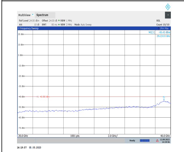
1-N48-PC3-30-40-L-1-DFT-PI2BPSK-Inner_1RB_Lef t-1@1-12000-20000-Ant1-17330.80--42.05--40-PAS
