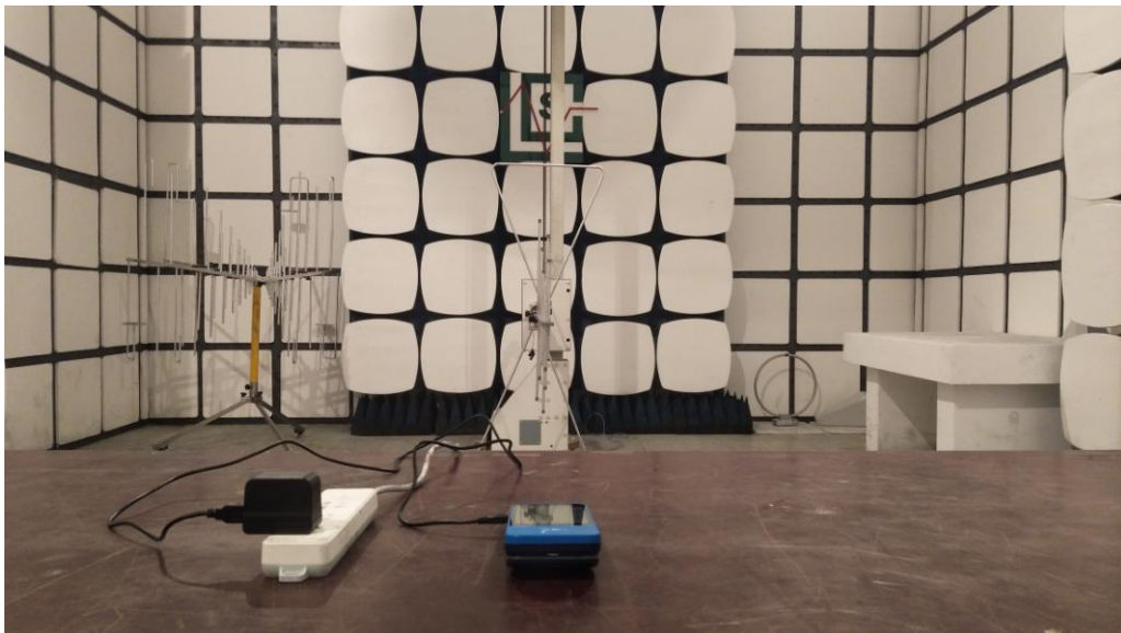
Fig. 2 (30MHz~1GHz)
