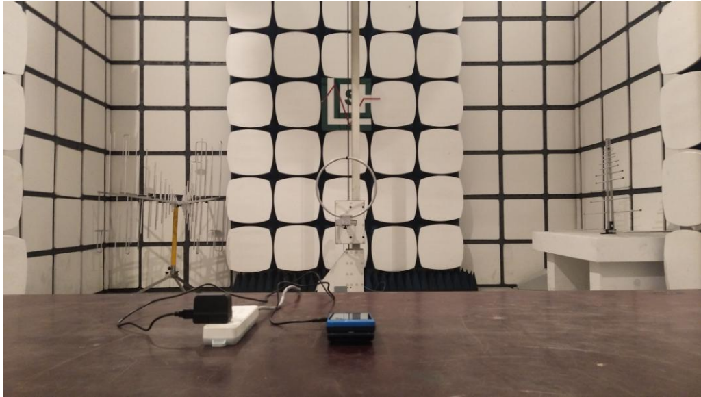
Fig. 1 (Below 30MHz)
