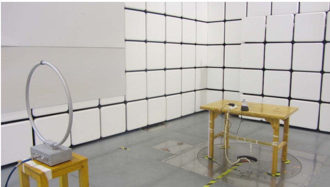
9kHz - 30MHz
