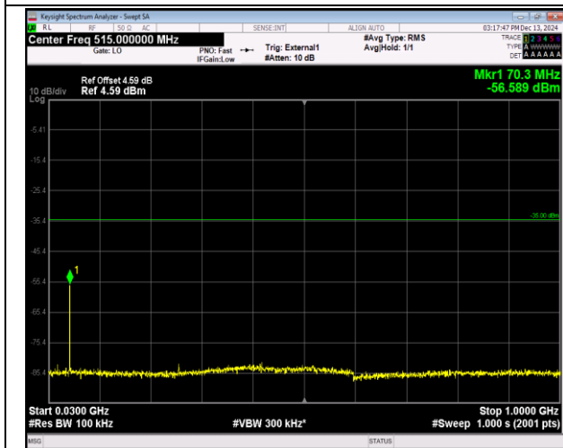
41(2555-2655)-41(2555-2655)-5MHz-20MHz-16QAM-16 QAM-41023-41140-1RB#0-ORB#0-30~1000MHz-PASS
