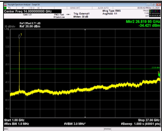
41(2555-2655)-41(2555-2655)-20MHz-5MHz-QPSK-QPSK- 40715-40832-1RB#0-1RB#24-1000~27000MHz-PASS
