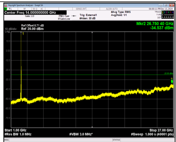
41(2555-2655)-41(2555-2655)-20MHz-5MHz-16QAM-16QA M-41090-41207-1RB#0-0RB#0-1000~27000MHz-PASS
