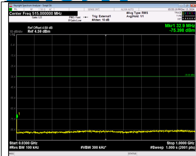
41(2555-2655)-41(2555-2655)-20MHz-5MHz-QPSK-QPS K-40715-40832-1RB#0-1RB#24-30~1000MHz-PASS
