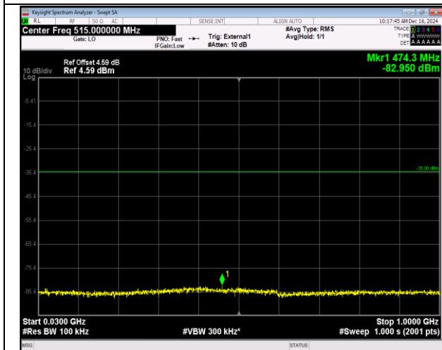
41(2555-2655)-41(2555-2655)-20MHz-20MHz-16QAM-16 QAM-40340-40538-1RB#0-0RB#0-30~1000MHz-PASS
