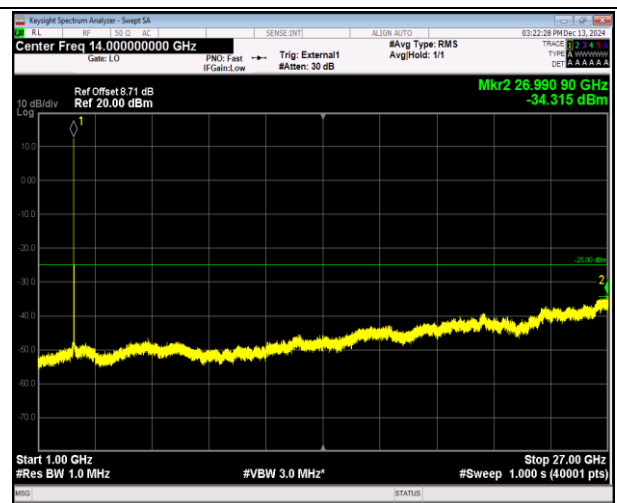
41(2555-2655)-41(2555-2655)-5MHz-20MHz-QPSK-QPSK- 41023-41140-25RB#0-100RB#0-1000~27000MHz-PASS
