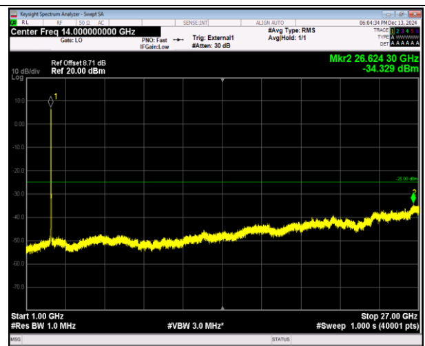
41(2555-2655)-41(2555-2655)-20MHz-5MHz-QPSK-QPSK- 41090-41207-100RB#0-25RB#0-1000~27000MHz-PASS
