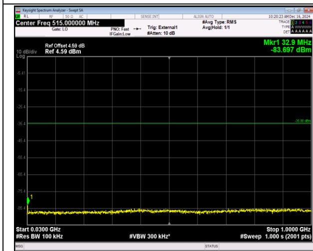
41(2555-2655)-41(2555-2655)-20MHz-20MHz-QPSK-QP SK-40340-40538-1RB#0-1RB#99-30~1000MHz-PASS
