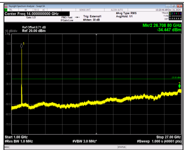
41(2555-2655)-41(2555-2655)-20MHz-20MHz-QPSK-QPS K-40340-40538-1RB#0-1RB#99-1000~27000MHz-PASS
