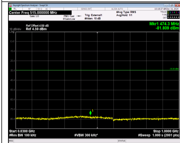
41(2555-2655)-41(2555-2655)-20MHz-20MHz-QPSK-QP SK-40340-40538-1RB#99-ORB#0-30~1000MHz-PASS
