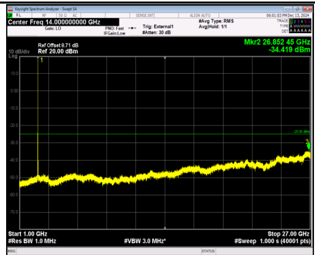
41(2555-2655)-41(2555-2655)-20MHz-5MHz-QPSK-QPSK- 41090-41207-1RB#99-0RB#0-1000~27000MHz-PASS
