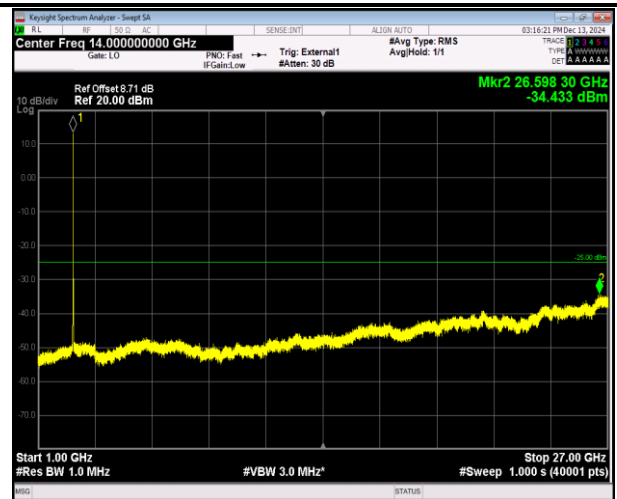
41(2555-2655)-41(2555-2655)-5MHz-20MHz-16QAM-16QAM-40648-40765-25RB#0-100RB#0-1000~27000MHz-PASS M
