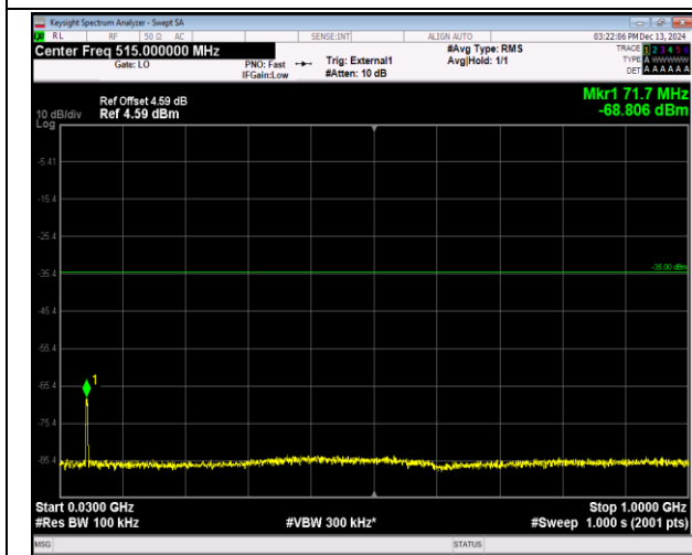
41(2555-2655)-41(2555-2655)-5MHz-20MHz-QPSK-QPS K-41023-41140-25RB#0-100RB#0-30~1000MHz-PASS
