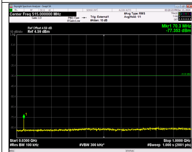
41(2555-2655)-41(2555-2655)-5MHz-20MHz-QPSK-QPSK-41023-41140-1RB#0-1RB#99-30~1000MHz-PASS K
