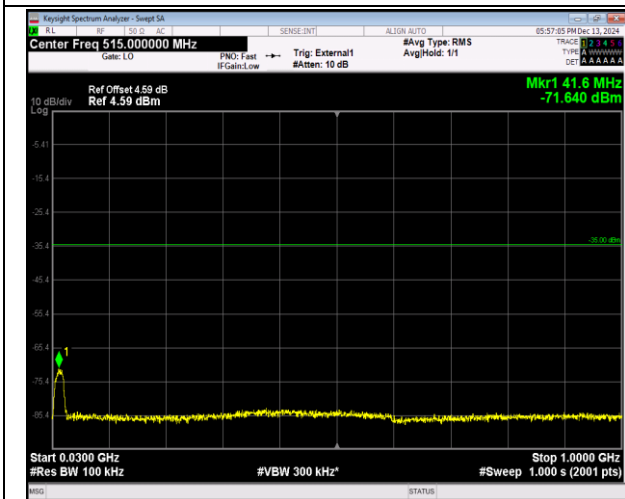
41(2555-2655)-41(2555-2655)-20MHz-5MHz-QPSK-QPS K-40715-40832-100RB#0-25RB#0-30~1000MHz-PASS
