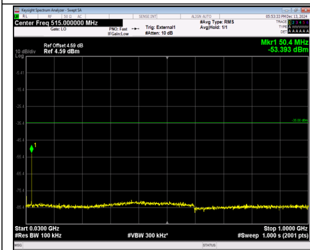
41(2555-2655)-41(2555-2655)-20MHz-5MHz-QPSK-QPS K-40715-40832-1RB#99-0RB#0-30~1000MHz-PASS
