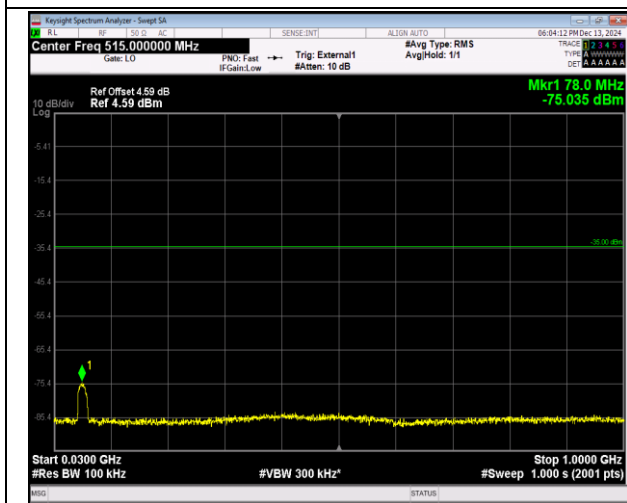
41(2555-2655)-41(2555-2655)-20MHz-5MHz-QPSK-QPSK K-41090-41207-100RB#0-25RB#0-30~1000MHz-PASS
