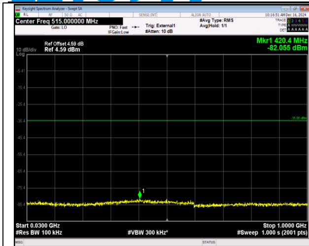
41(2555-2655)-41(2555-2655)-20MHz-20MHz-QPSK-QP SK-40340-40538-1RB#0-ORB#0-30~1000MHz-PASS
