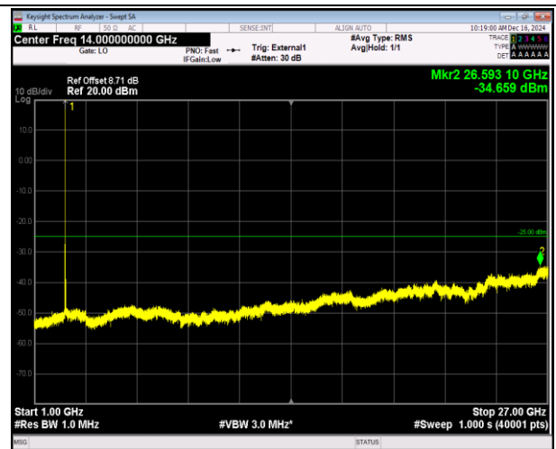
41(2555-2655)-41(2555-2655)-20MHz-20MHz-QPSK-QPS K-40340-40538-1RB#99-ORB#0-1000~27000MHz-PASS
