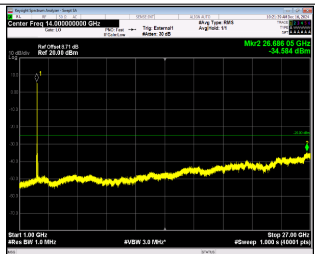
41(2555-2655)-41(2555-2655)-20MHz-20MHz-16QAM-16Q AM-40340-40538-1RB#0-1RB#99-1000~27000MHz-PASS
