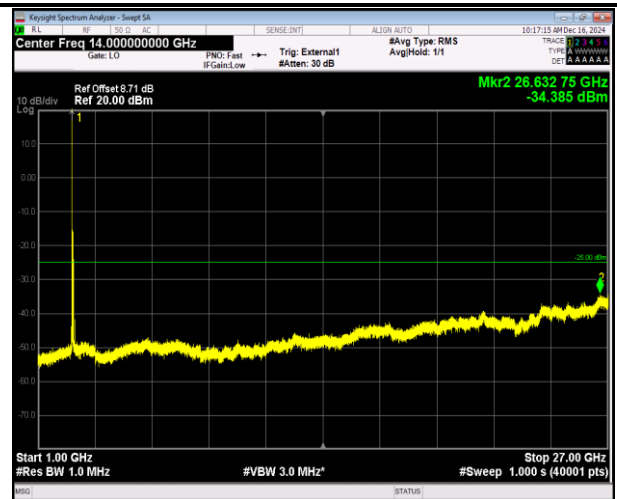
41(2555-2655)-41(2555-2655)-20MHz-20MHz-QPSK-QPS K-40340-40538-1RB#0-ORB#0-1000~27000MHz-PASS
