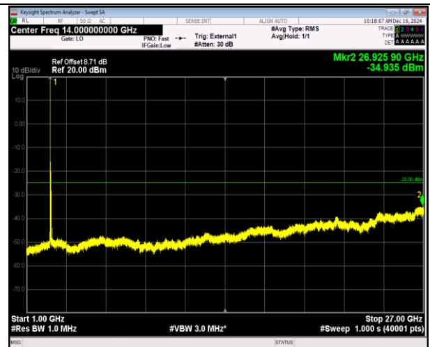
41(2555-2655)-41(2555-2655)-20MHz-20MHz-16QAM-16Q AM-40340-40538-1RB#0-0RB#0-1000~27000MHz-PASS
