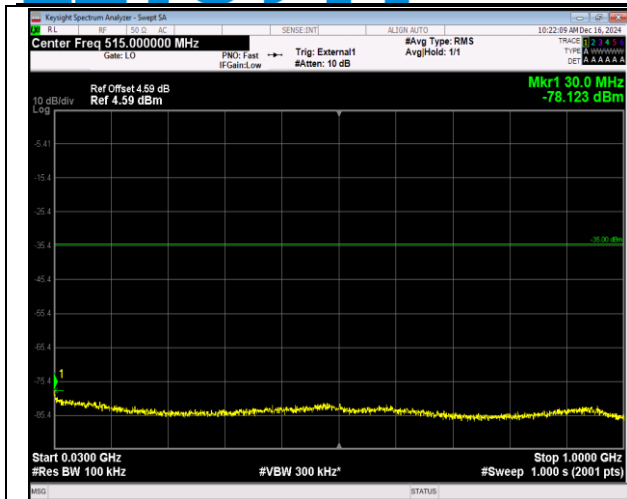
41(2555-2655)-41(2555-2655)-20MHz-20MHz-QPSK-QP SK-40340-40538-100RB#0-100RB#0-30~1000MHz-PAS S
