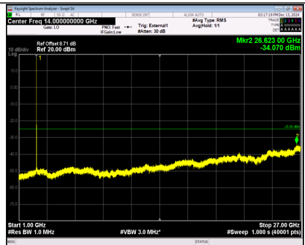
41(2555-2655)-41(2555-2655)-5MHz-20MHz-QPSK-QPSK-41023-41140-1RB#0-0RB#0-1000~27000MHz-PASS K
