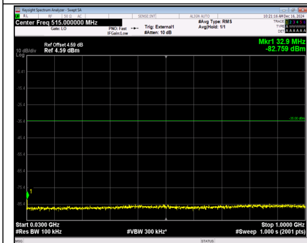
41(2555-2655)-41(2555-2655)-20MHz-20MHz-16QAM-16 QAM-40340-40538-1RB#0-1RB#99-30~1000MHz-PASS
