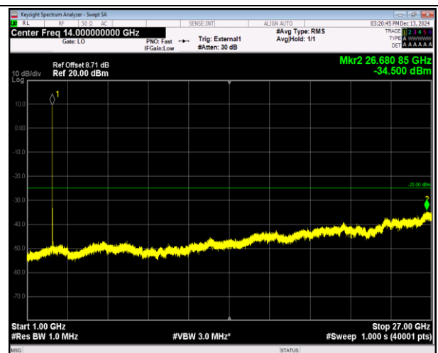
41(2555-2655)-41(2555-2655)-5MHz-20MHz-QPSK-QPSK-41023-41140-1RB#0-1RB#99-1000~27000MHz-PASS K
