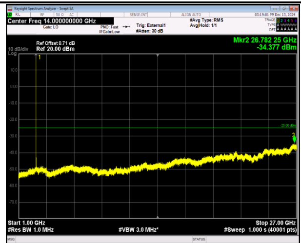
41(2555-2655)-41(2555-2655)-5MHz-20MHz-QPSK-QPSK- 41023-41140-1RB#24-ORB#0-1000~27000MHz-PASS
