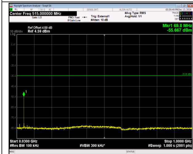
41(2555-2655)-41(2555-2655)-20MHz-5MHz-16QAM-16 QAM-41090-41207-1RB#0-0RB#0-30~1000MHz-PASS
