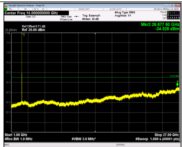
41(2555-2655)-41(2555-2655)-5MHz-20MHz-16QAM-16QA M-41023-41140-1RB#0-ORB#0-1000~27000MHz-PASS
