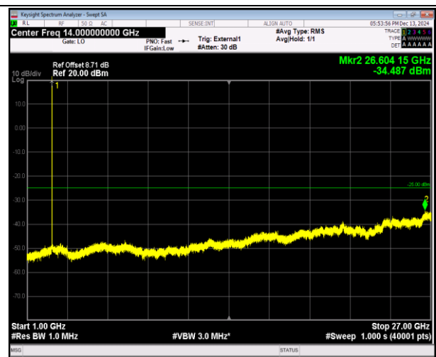
41(2555-2655)-41(2555-2655)-20MHz-5MHz-QPSK-QPSK- 40715-40832-1RB#99-0RB#0-1000~27000MHz-PASS
