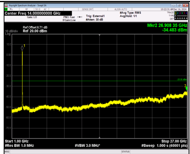
41(2555-2655)-41(2555-2655)-20MHz-20MHz-QPSK-QPS K-40340-40538-100RB#0-100RB#0-1000~27000MHz-PAS S
