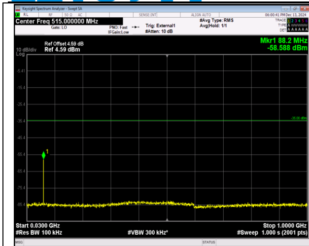
41(2555-2655)-41(2555-2655)-20MHz-5MHz-QPSK-QPSK K-41090-41207-1RB#99-0RB#0-30~1000MHz-PASS
