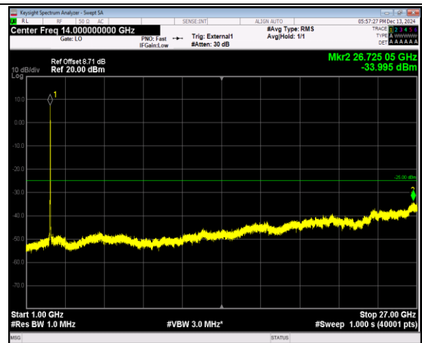
41(2555-2655)-41(2555-2655)-20MHz-5MHz-QPSK-QPSK- 40715-40832-100RB#0-25RB#0-1000~27000MHz-PASS
