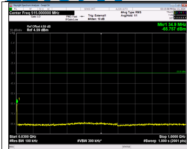
41(2555-2655)-41(2555-2655)-5MHz-20MHz-16QAM-16QAM-40648-40765-25RB#0-100RB#0-30~1000MHz-PAS S
