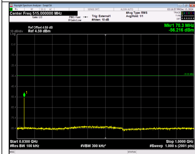
41(2555-2655)-41(2555-2655)-5MHz-20MHz-QPSK-QPSK-41023-41140-1RB#0-0RB#0-30~1000MHz-PASS K
