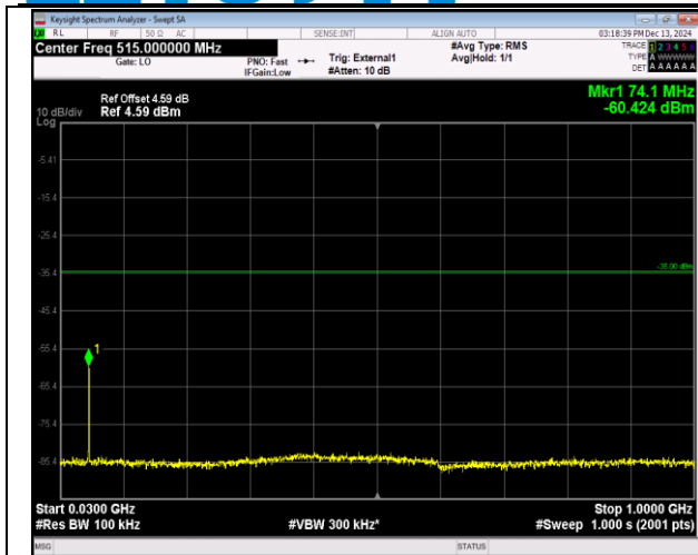
41(2555-2655)-41(2555-2655)-5MHz-20MHz-QPSK-QPS K-41023-41140-1RB#24-ORB#0-30~1000MHz-PASS
